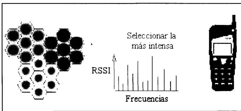
Figura 1-5.- Rastreo de las frecuencias del canal de control
