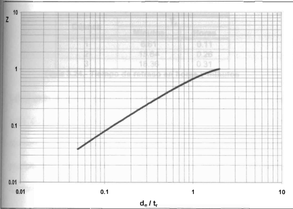
Figura 3.10.- Factor de reducción en función del tiempo de retraso y la duración en exceso
