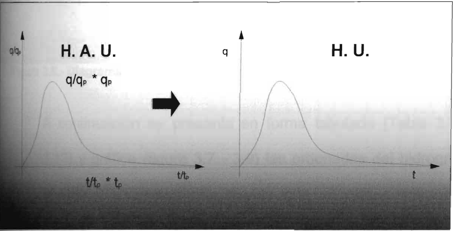
Figura 3.5.- Diagrama del cálculo del hidrograma unitario
