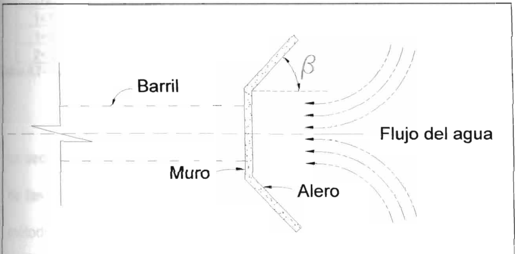
Figura 4.4.- Ángulo de alabeo [b]
