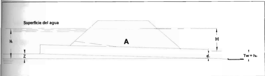
Figura 4.2.- Alcantarilla estándar- Flujo a superficie libre
