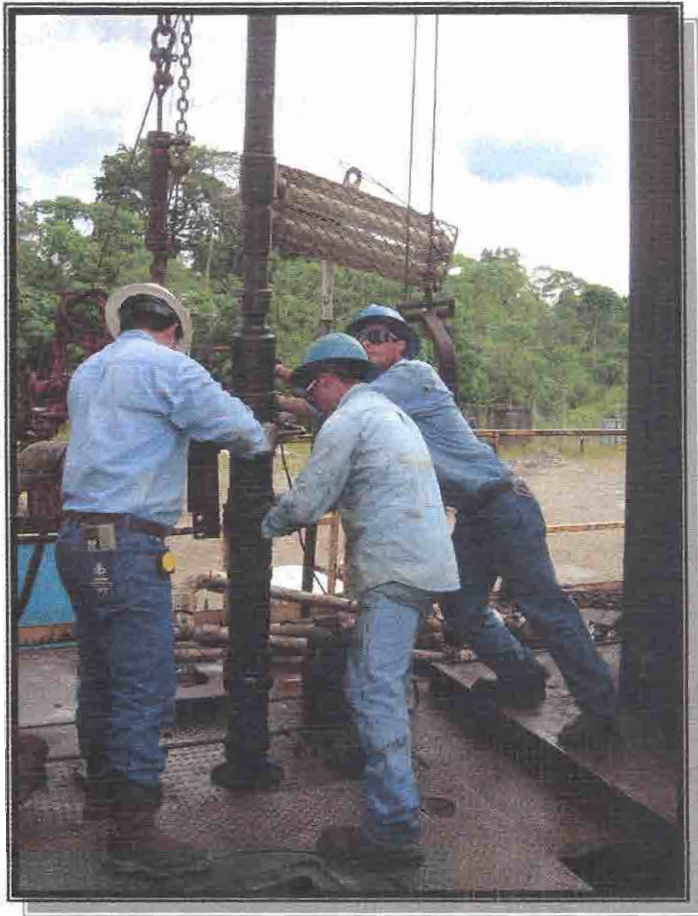
Foto No.12 Armando BHA de evaluación, Angel Navarrete O. Enero 2008.
