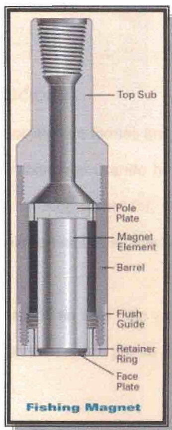
Figura 23. "Fishing Magnet", fuente: Internet.
