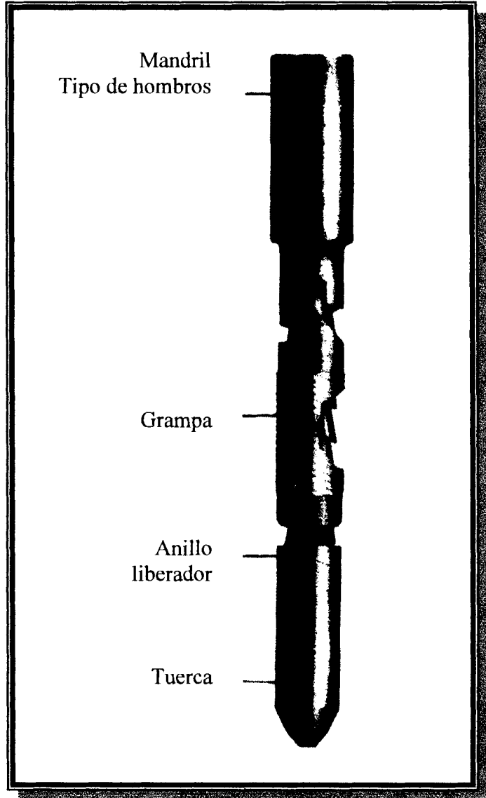
Figura 1. "Releasing Spear" tipo de hombros; fuente: Bowen Fishing tools Technical Manual No.2300.
