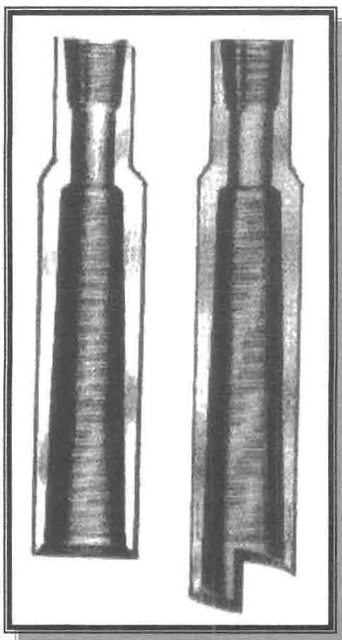
Figura 16. Die Collars tipo "A" y tipo "B", fuente: Bowen Fishing tools Technical Manual No.2100
