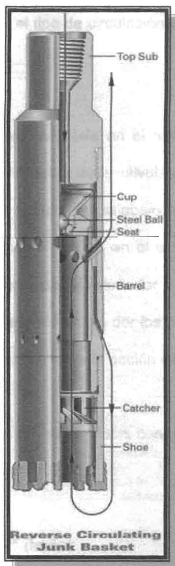
Figura 22. Canasta con Circulación Inversa, fuente: Internet.
