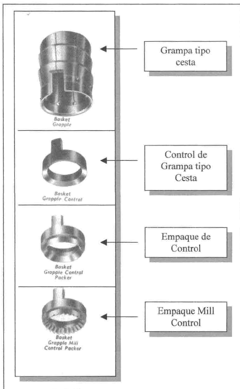
Figura 12. Grampa tipo cesta y empaques, fuente: Bowen Fishing Tools Technical Manual No.1150
