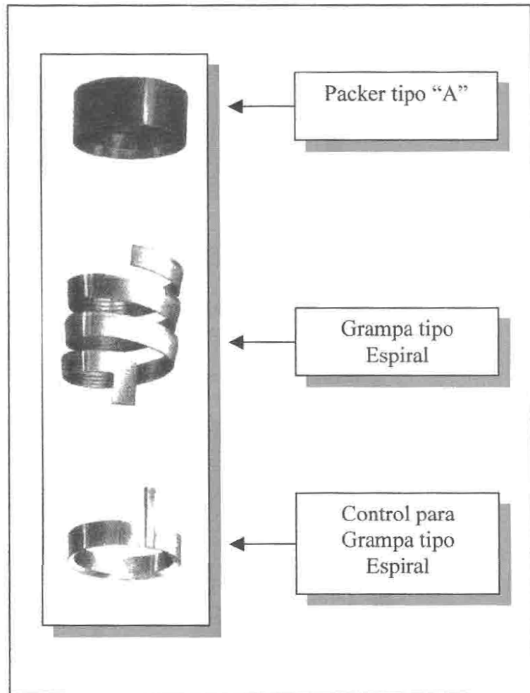
Figura 13. Grampa tipo espiral, empaque y guía fuente: Bowen Fishing tools Technical Manual No.1150.
