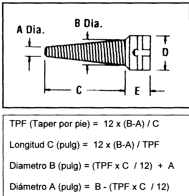
Figura 8. Gráfico del Taper Tap y fórmulas, fuente: Bowen Fishing tools Technical Manual No.2100.
