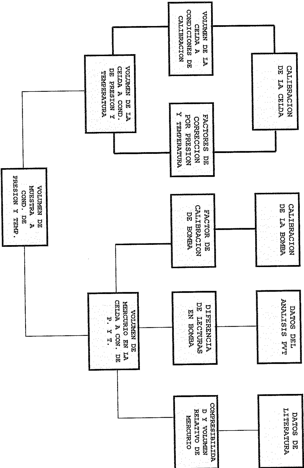
Fig. 6.1 CALCULO DE LOS VOLUMENES DE LA MUESTRA A CONDICIONES DE YACIMIENTO
