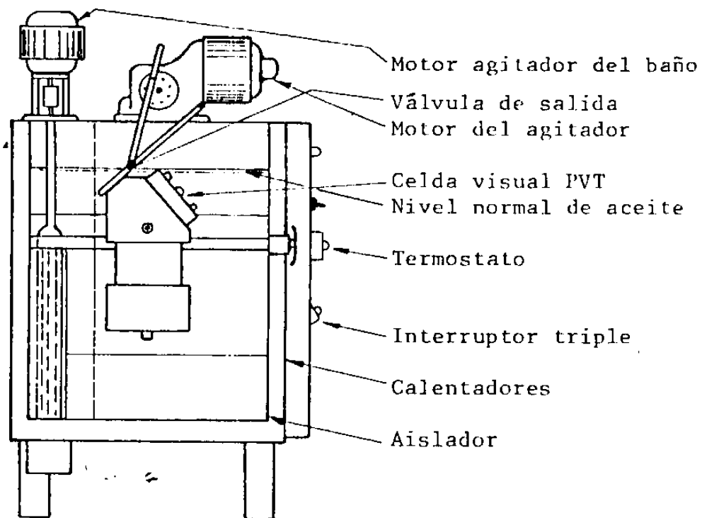
Fig. No 2.2 PARTES Y COMPONENTES DE LA CELDA PVT
