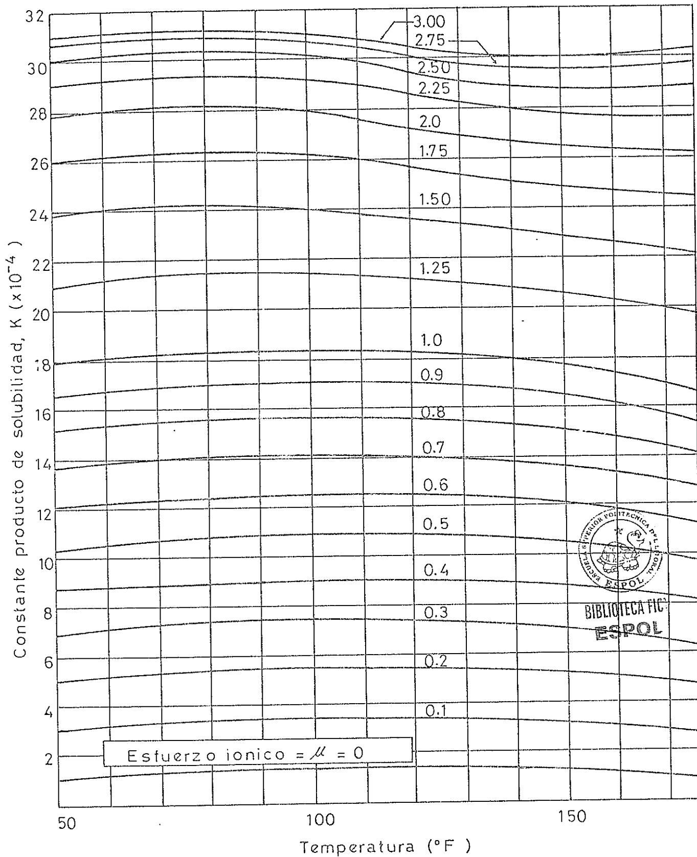
FIG. 8 Determinación de la constante producto de solubilidad del sulfato de calcio(yeso).
