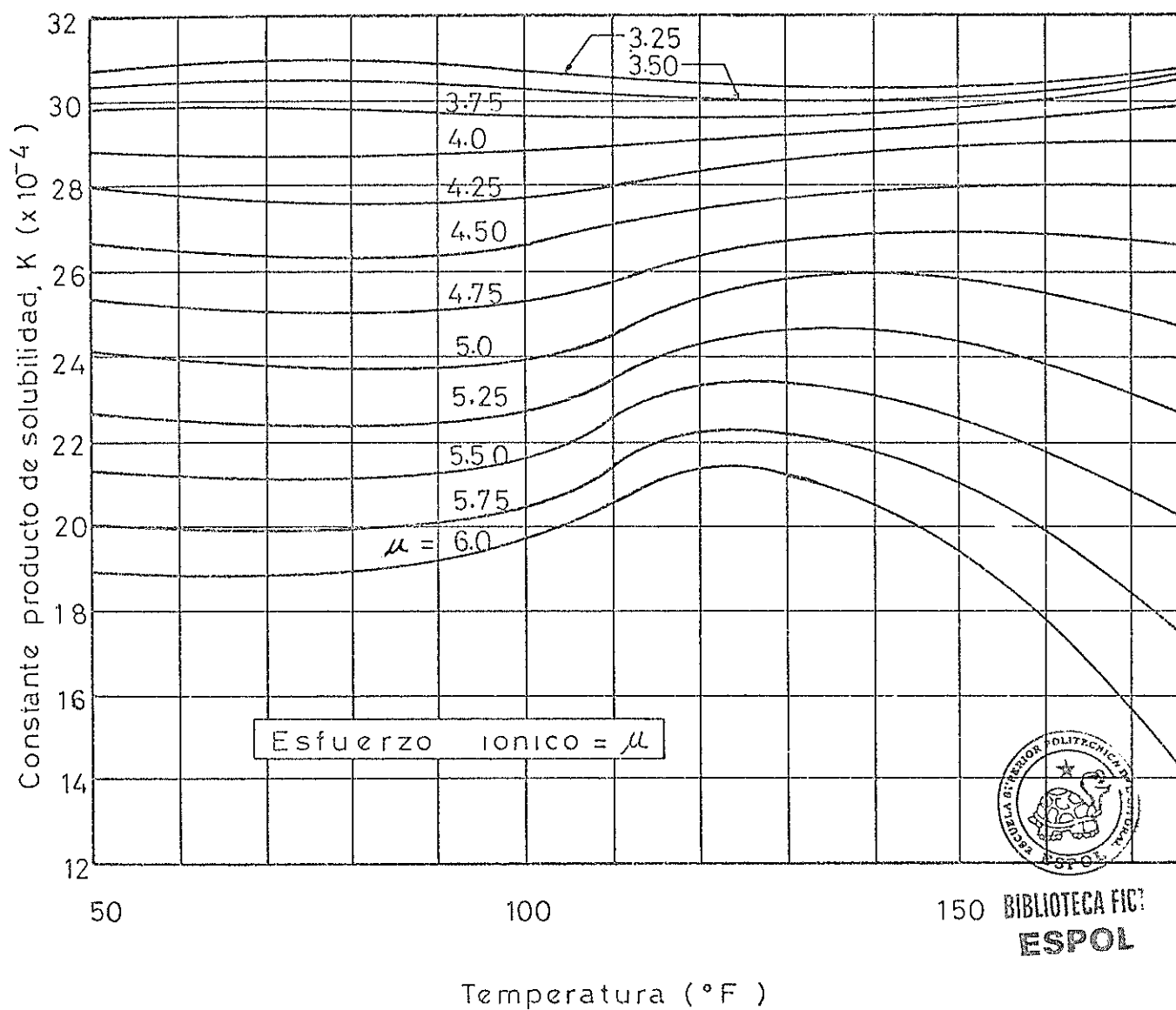
FIG. 9. Determinación de la constante producto de solubilidad del carbonato de calcio.
