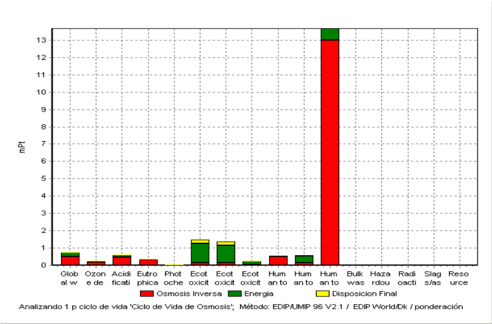
FIGURA 3.22. PONDERACIÓN EDIP 96
