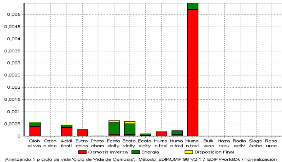
FIGURA 3.21. NORMALIZACIÓN EDIP 96
