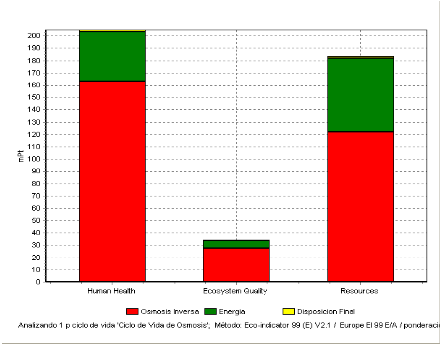
FIGURA 3.9. PONDERACIÓN ECO-INDICATOR 99
