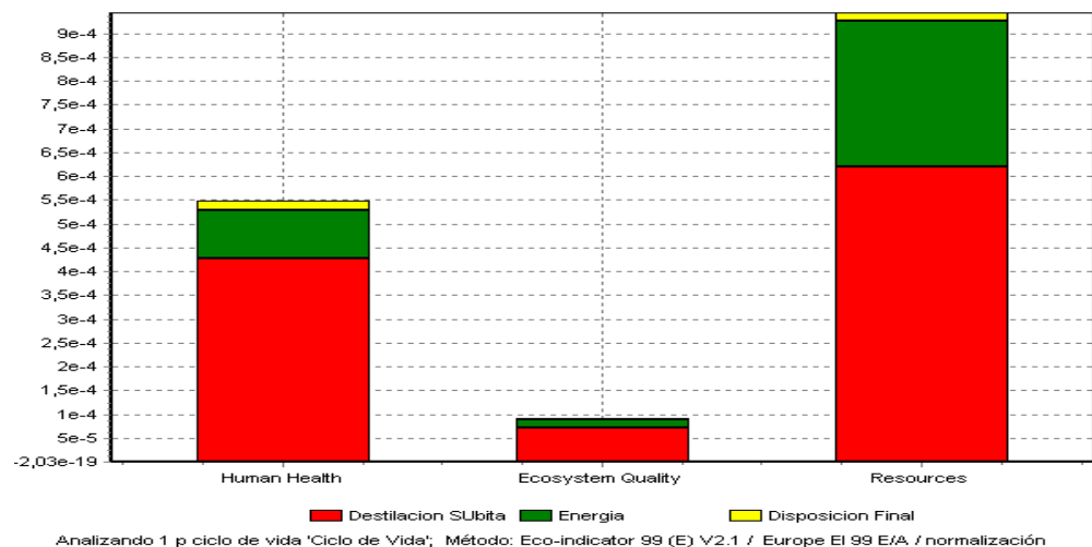
FIGURA 3.12. NORMALIZACIÓN ECO-INDICATOR 99
