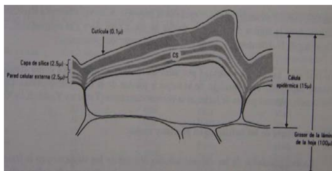
Gráfico 1.2 Esquema de una célula epidérmica de la hoja de la planta de arroz, CS=celulosa silicada (8) (18)
