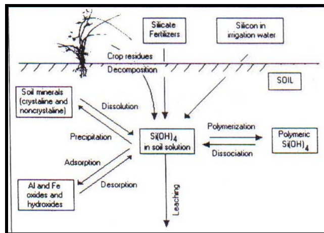
Gráfico 1. 1 Principales procesos y transformaciones que afectan la concentración del silicio en la solución del suelo (18).
