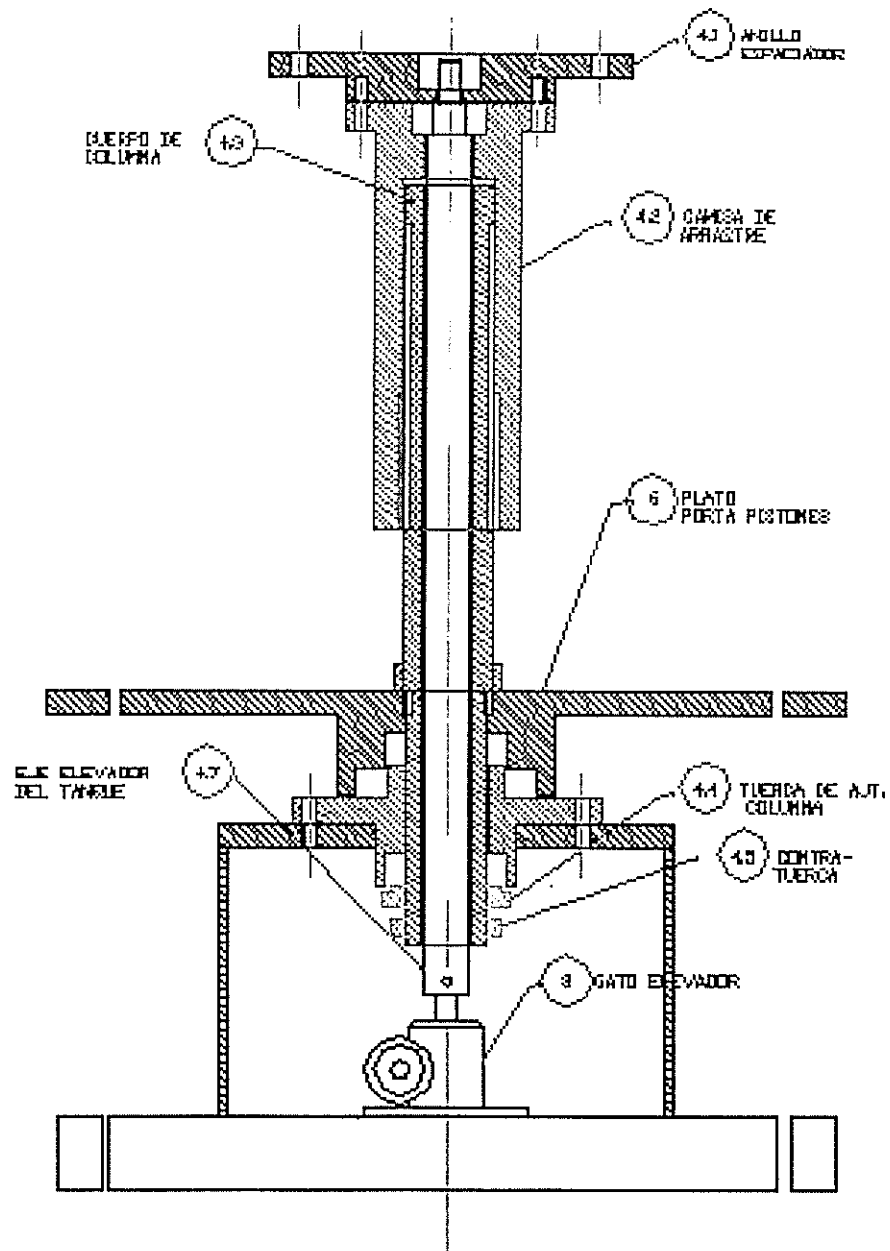
FIGURA 20. COLUMNA CENTRAL ( 4 )
