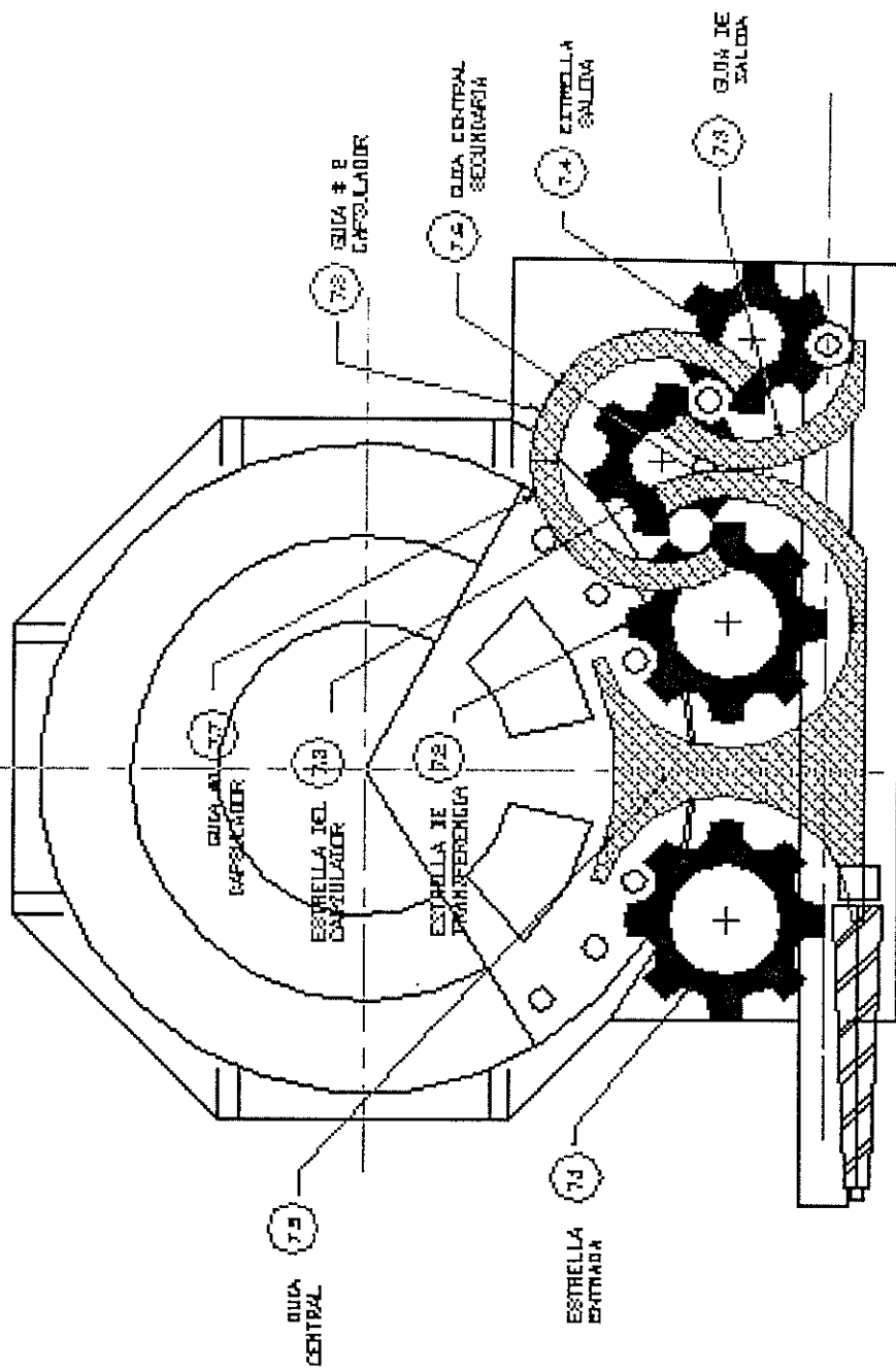
FIGURA 21. JUEGO DE MANEJO DE BOTELLAS ( 7 )
