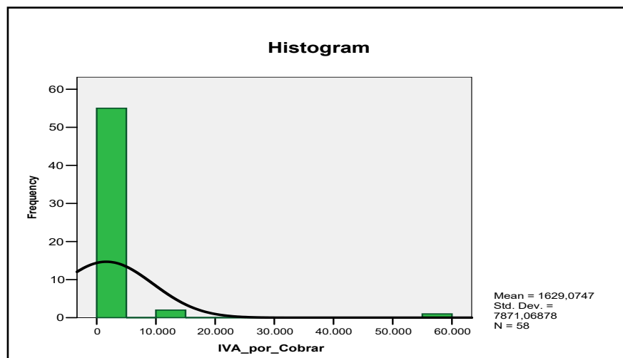
Figura 3.2.1.4 Histograma (Saldos CxC-IVA)
