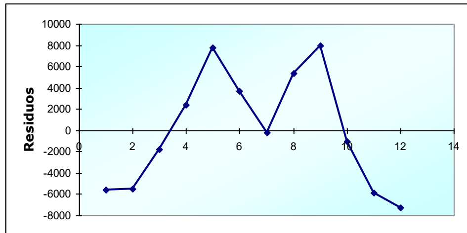
Figura 3.2.1.5: Error Estándar de Estimación
