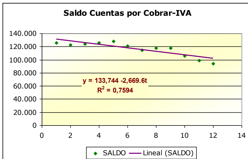
Figura 3.2.1.5 Línea de Tendencia (Saldos CxC-IVA)
