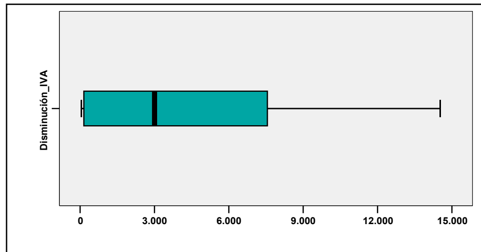
Figura 3.2.1.2 Diagrama de cajas (IVA recuperado)
