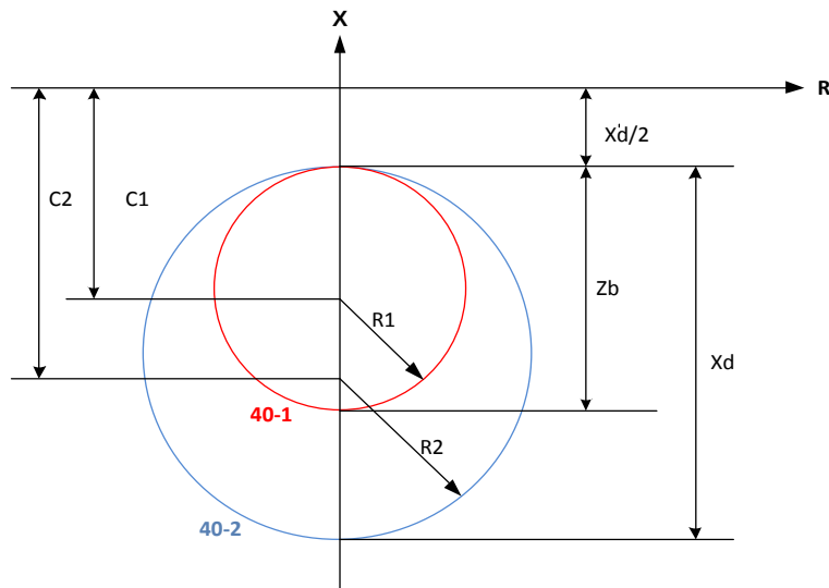
Fig. 3.3.6.2: Características mho
