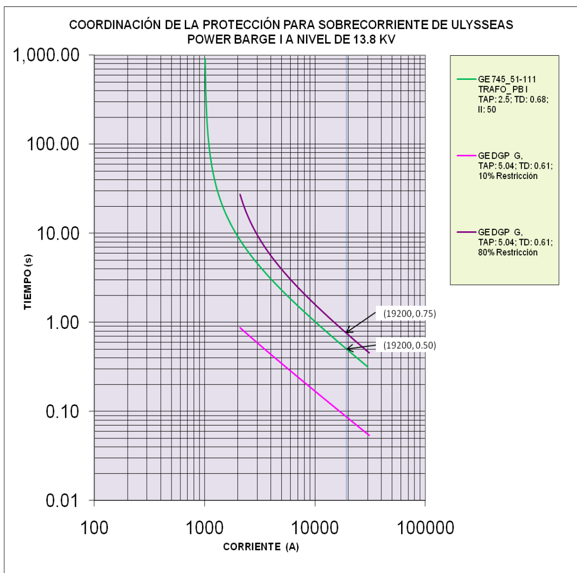
gráfica b: Coordinación de la protección para sobrecorriente en Ulyss Power Barge 1 a nivel de 13.8KV
