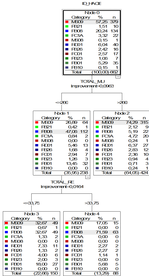
Figura 3.2 Árbol de decisiones – Algoritmo C&RT
