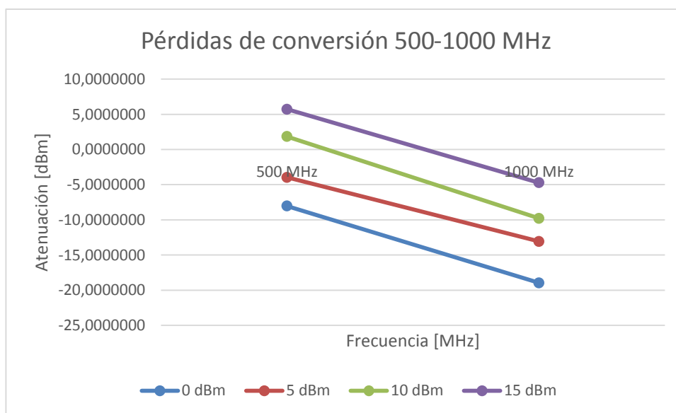
Figura 3.13: Pérdidas de conversión 500-1000 MHz.
