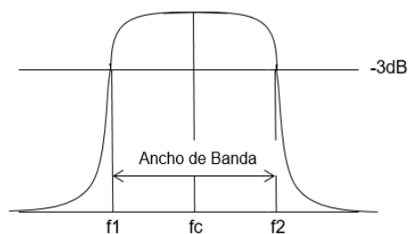
Figura 2.7: Ancho de banda.
