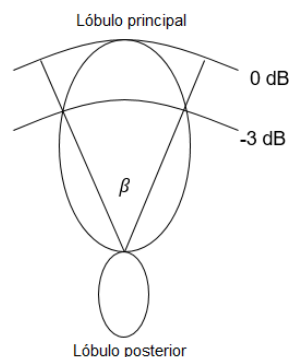
Figura 2.8: Ancho de haz de una antena.
