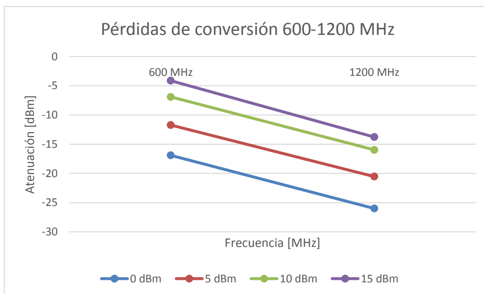
Figura 3.15: Pérdidas de conversión 600-1200 MHz.
