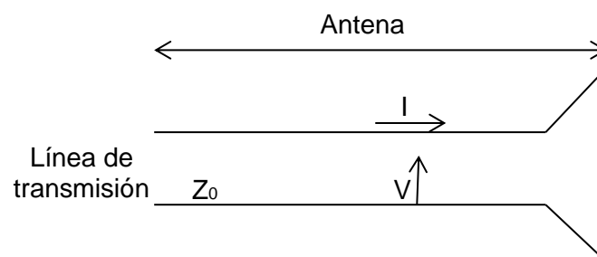
Figura 2.6: Impedancia de entrada de una antena.
