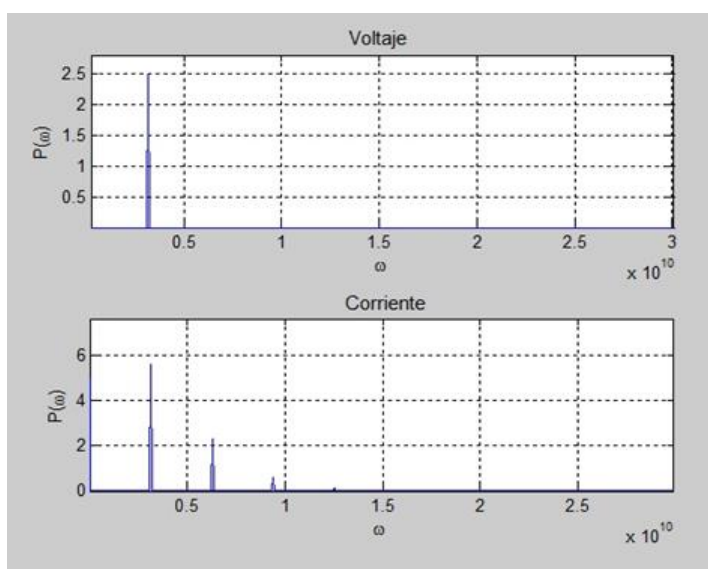
Figura 3.10: frecuencias fundamental y armónica.
