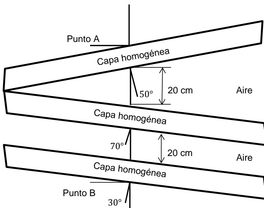
Figura 3.4: Escombros, modelo B.
