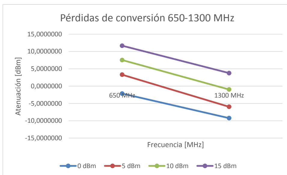
Figura 3.16: Pérdidas de conversión 650-1300 MHz.
