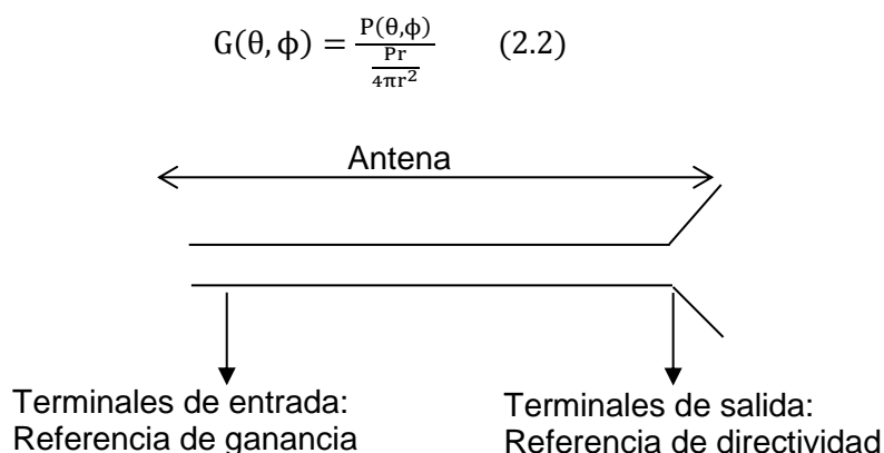
Figura 2.4: Ganancia y directividad en los terminales de una antena.
