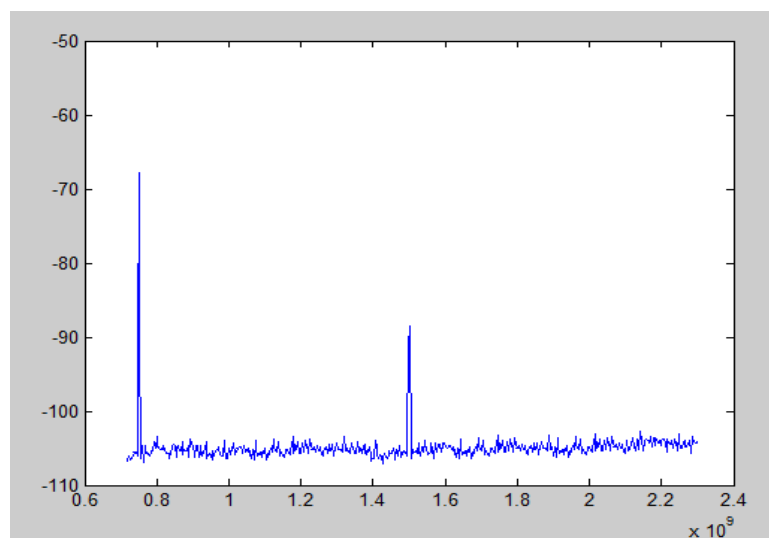
Figura 3.34: Frecuencias retransmitidas por el transpondedor en el ensayo.
