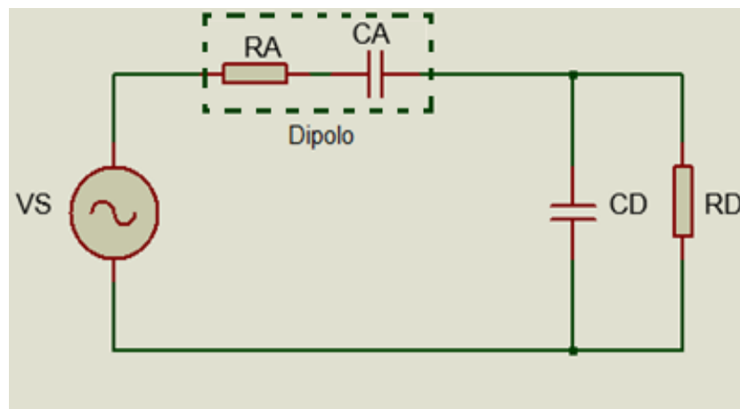
Figura 3.24: Equivalente Thévenin dipolo-diodo.
