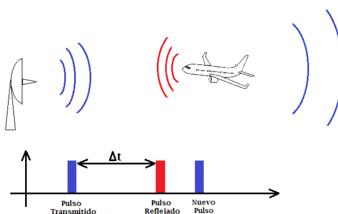
Figura 2.1: Principio del radar pulsado.
