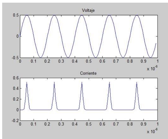
Figura 3.9: Señales de voltaje y corriente a través de un diodo schottky.
