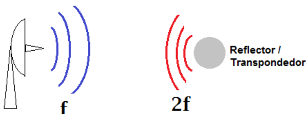
Figura 2.2: Detección de frecuencias armónicas.
