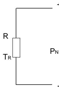
Figura 2.10: Potencia de ruido de una resistencia.
