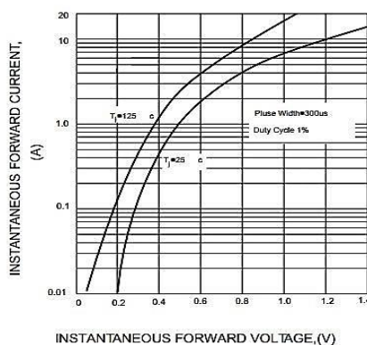
Figura 3.8: Relación no lineal del voltaje y corriente en el diodo BAT43. [21]
