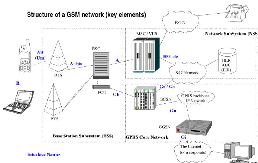
Figura 2.1. Esquema general de un sistema GSM [11]
