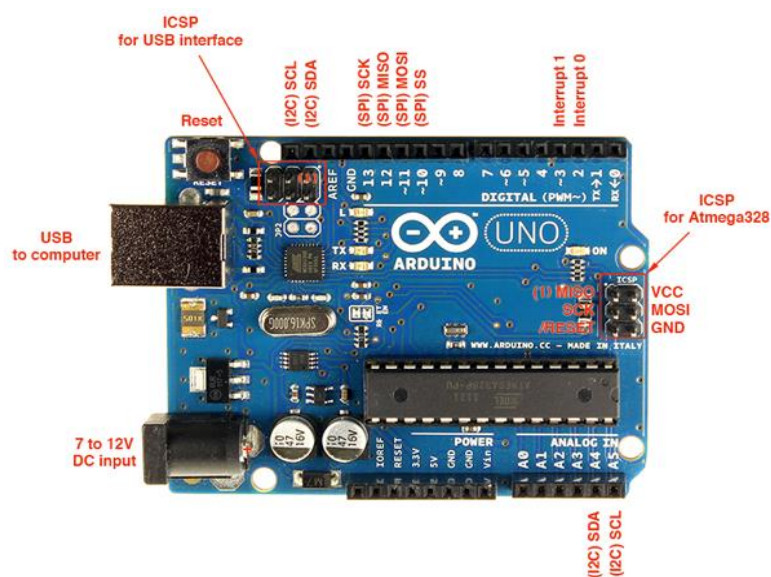
Figura 2.2. Placa Arduino [3]
