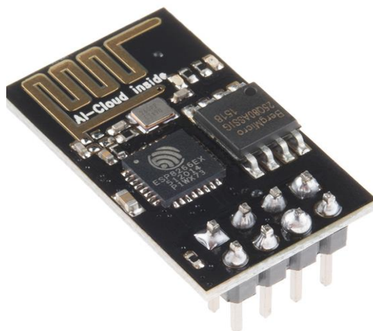
Figura 2.3. Módulo WIFI-ESP8266 [4]
