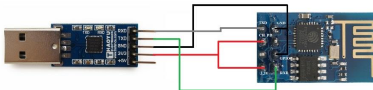
Figura 3.5. Conexión del Módulo ESP8266.
