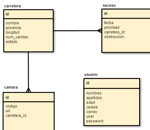
Figura 3.2. Diagrama Entidad-Relación.
