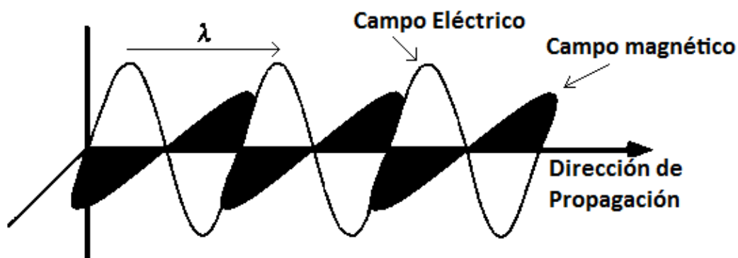
Figura 0.1. Onda Electromagnética
