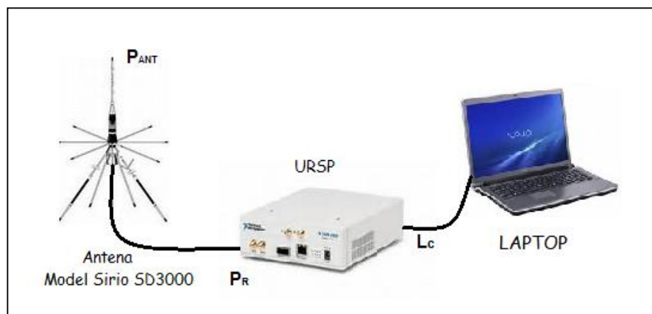
Fig.3.2: Sistema de medición implementado
