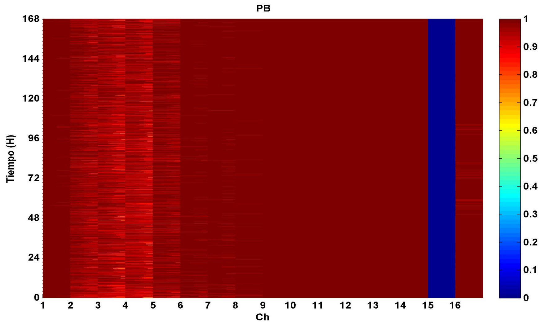
Figura 4.11: Disponibilidad de canales en la Planta Baja
