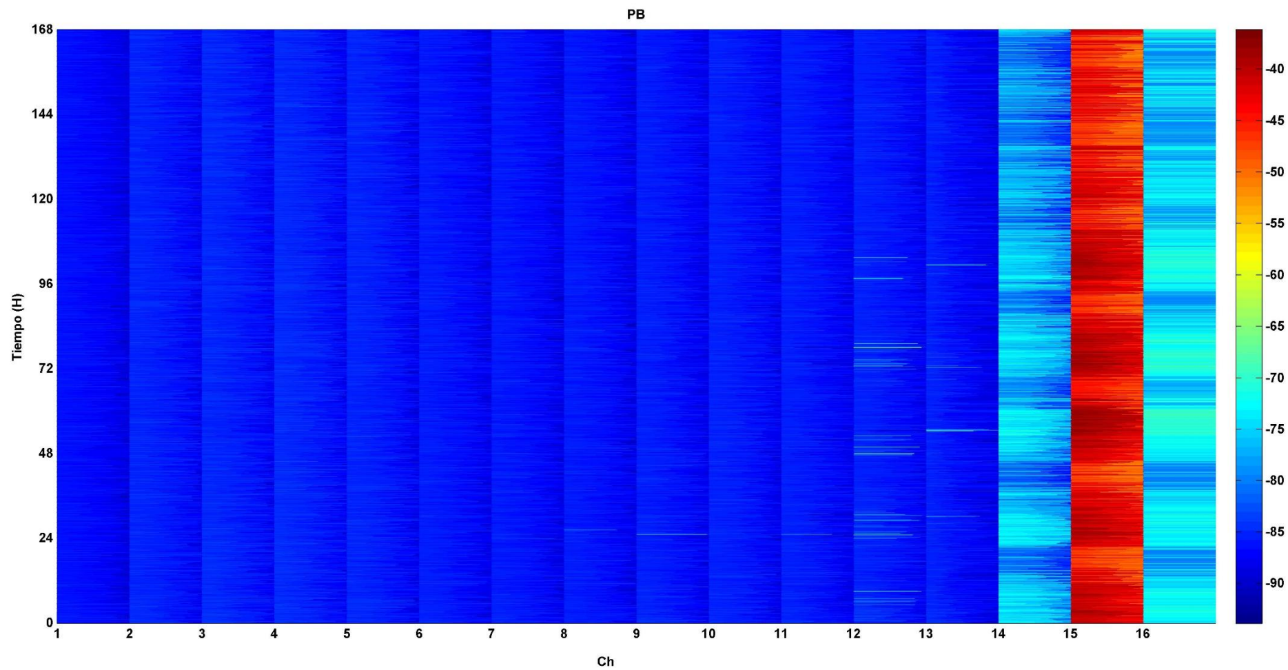
Figura 4.8: Niveles de Potencia en la Planta Baja
