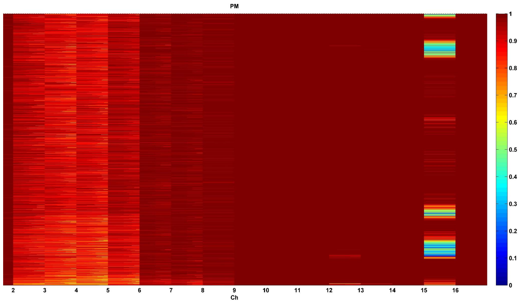
Figura 4.12: Disponibilidad de canales en la Planta media
