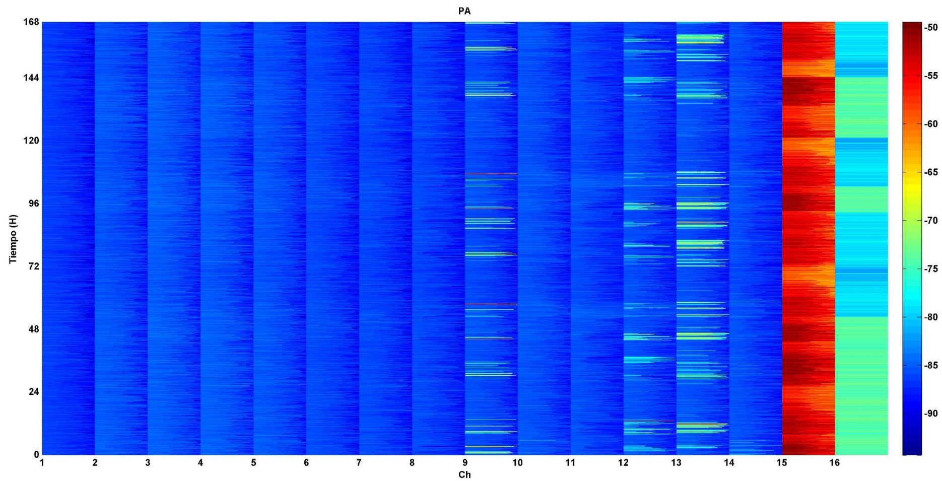
Figura 4.10: Niveles de Potencia en la Planta Alta
