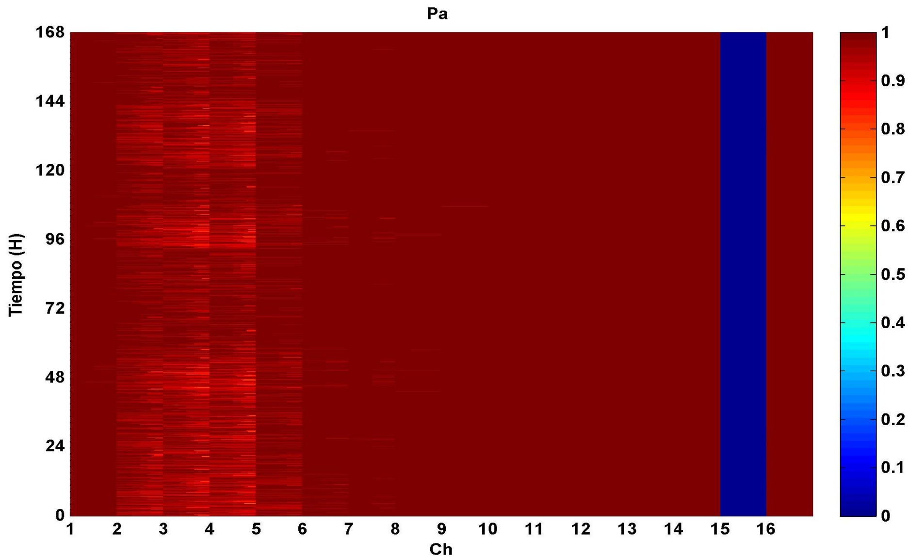
Figura 4.13: Disponibilidad de canales en la Planta Alta
