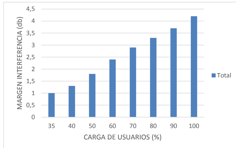
Figura 3.6: Margen de Interferencia en función a la carga de Usuarios
