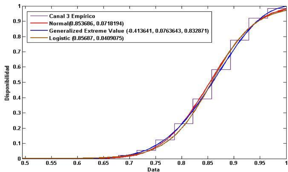
Figura 4.15: Modelamiento de canal correspondiente a la banda AWS
