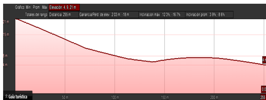
Fig. 4.2: Perfil de elevación en referencia a la Estación superior
