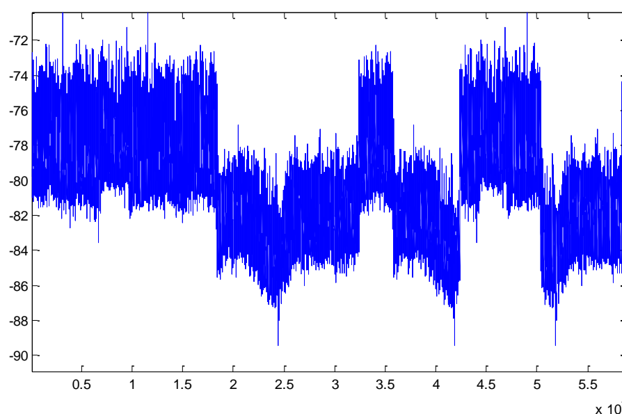
Figura 4.7: Niveles de Potencia recibidos en canal 16 de la Planta Alta
