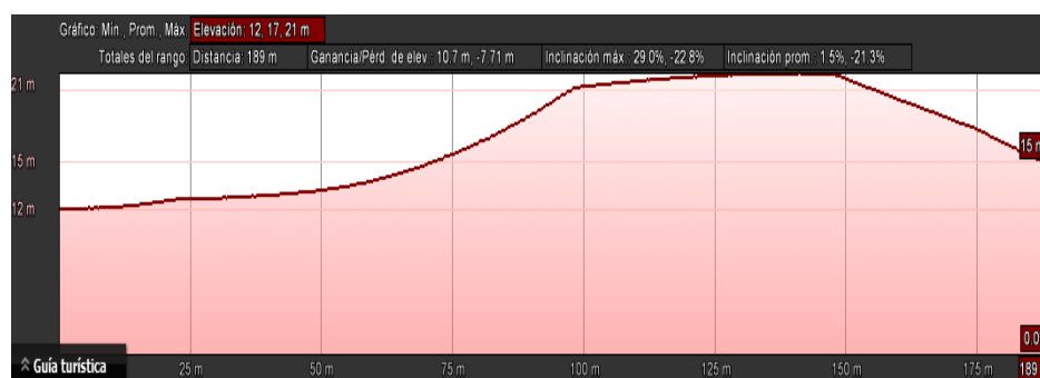
Fig. 4.3: Perfil de elevación en referencia a base inferior
