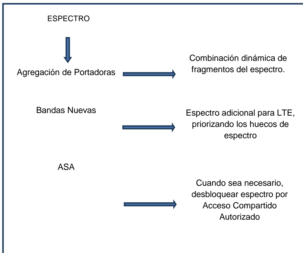
Figura 2.5: Maximización del espectro para mejorar la conectividad
