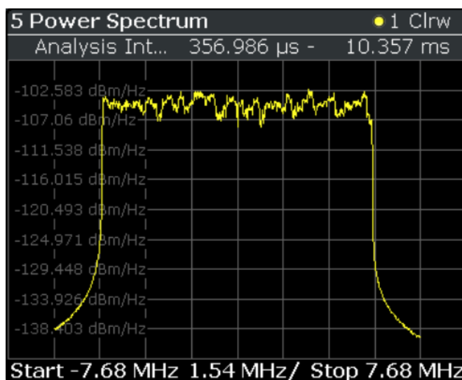
Figura 2.9: Ilustración de una Portadora de LTE, enlace de bajada
