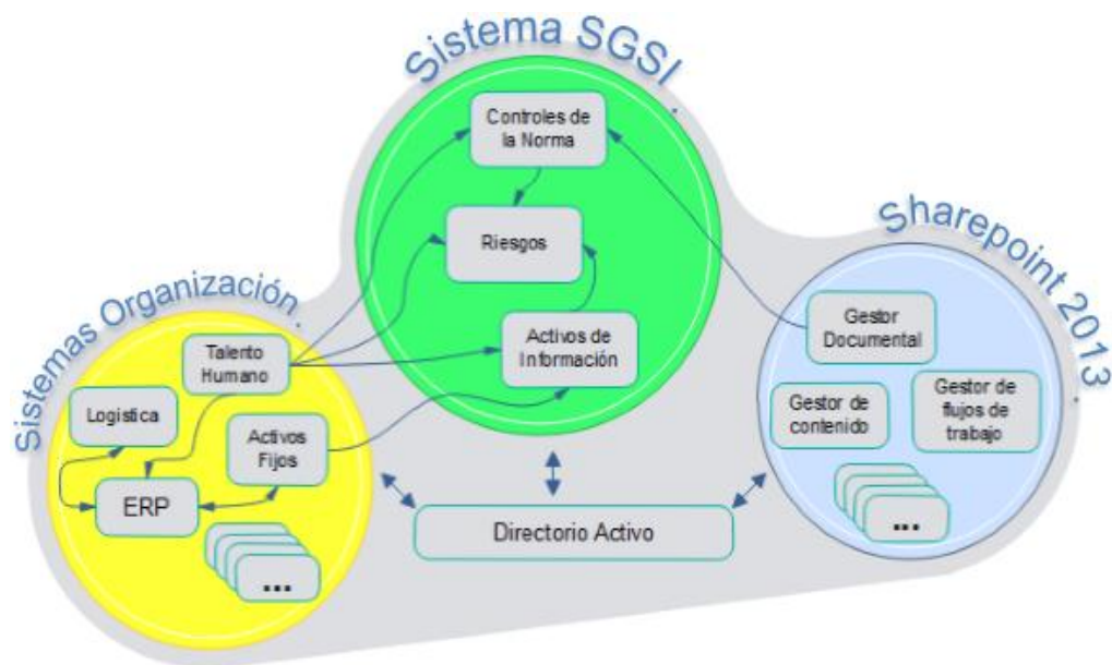
Figura 4.8 Diagrama de sistemas y subsistemas
