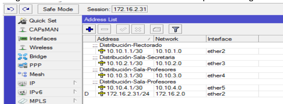
Figura 1.12 Asignación de redes
