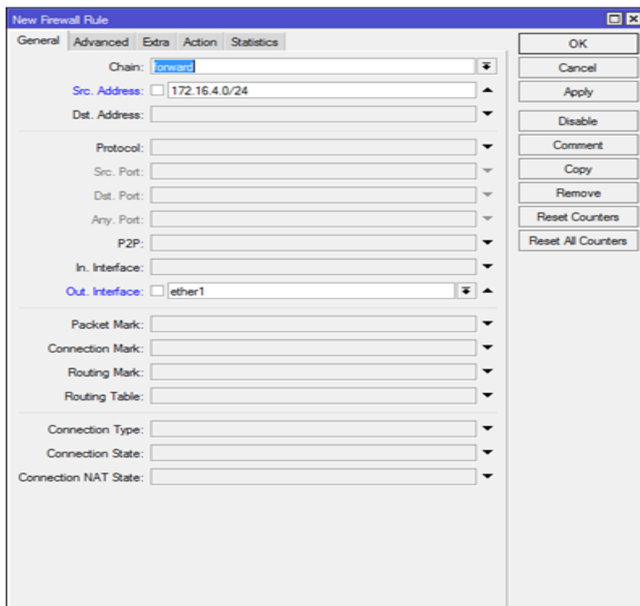
Figura 1.9 Bloqueo por contenido
