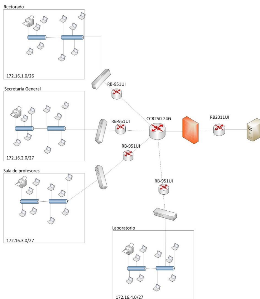
Figura 1.4 Esquema de la red en la Unidad Educativa
