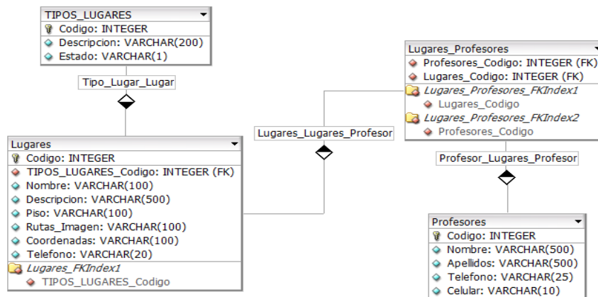
Figura 3.22 Modelo de Base de Datos
