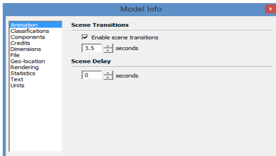
Figura 3.18 Configuración escenas
