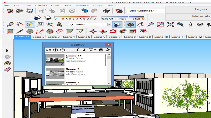
Figura 3.19 Agregar Escenas
