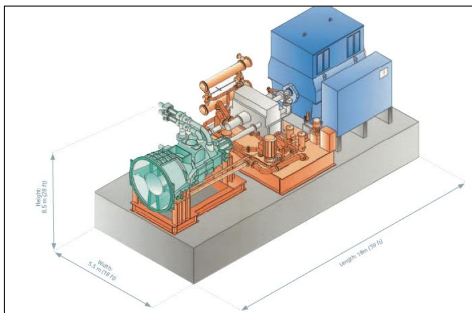
Figura 3.2: Diseño de turbina Siemens SST-400 GEO size 1.
