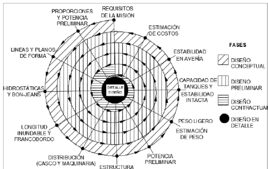
Figura No. 1.- Espiral de Diseño
