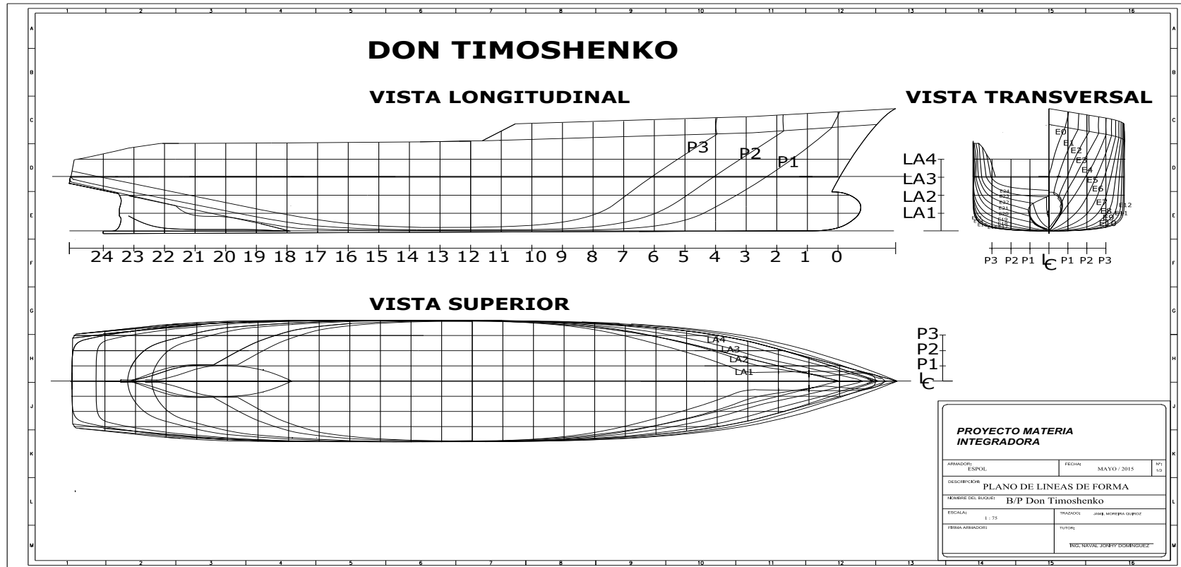
Figura No. 15.- Plano de Formas del Buque DON TIMOSHENKO
