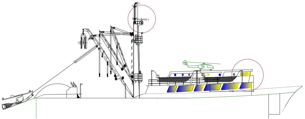
Figura 6.- Zonas de análisis de aceleración vertical
