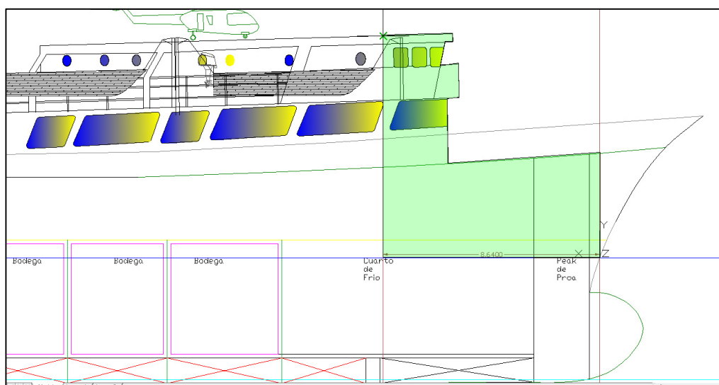
Figura No. 19.- Reserva de flotabilidad, buque proyecto
