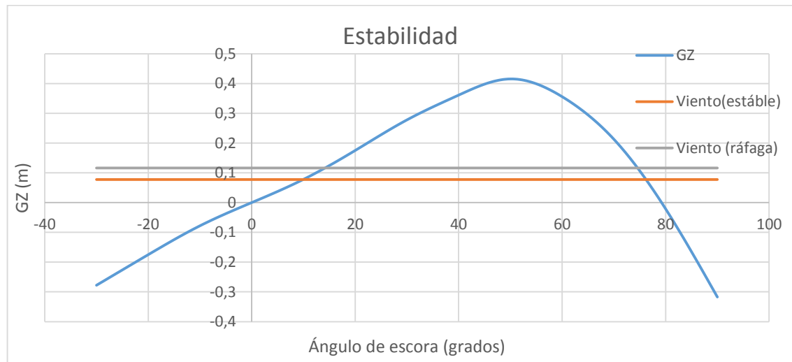
Figura No. 22.- Curva de Brazo Adrizante
