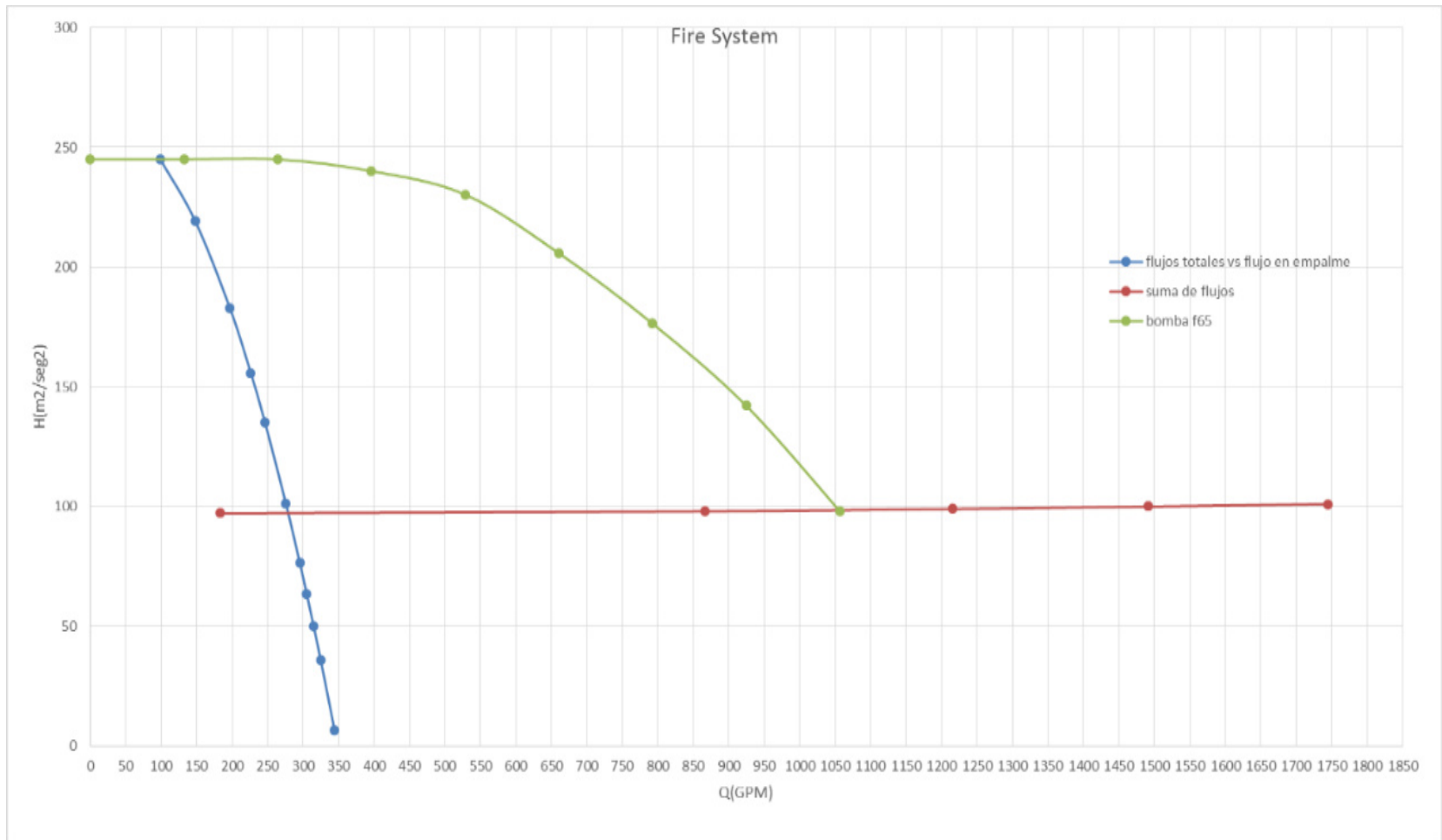
Figura No. 53.- Suma de Cabezales en serie
