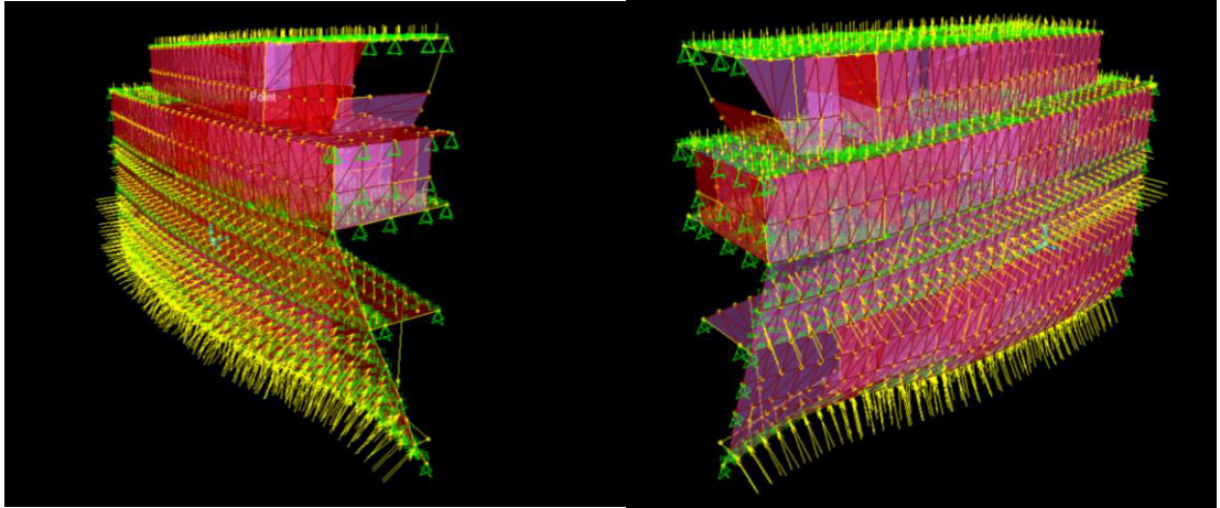
Figura No. 71.- Distribución de presiones en la estructura del Buque
