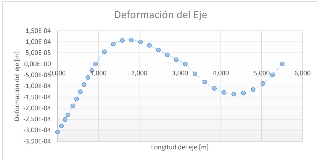
Figura No. 97.- Deformación del eje propulsor
