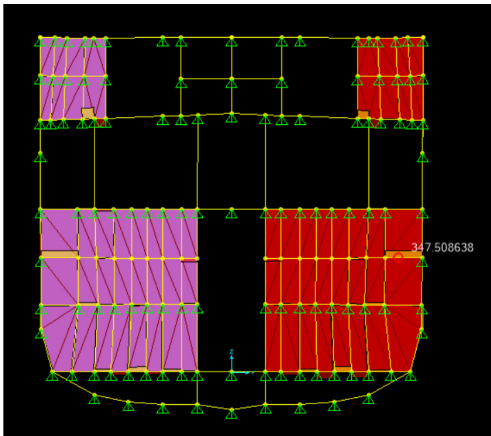
Figura No. 78.-Esfuerzo sobre vigas de cuadernas Maestra
