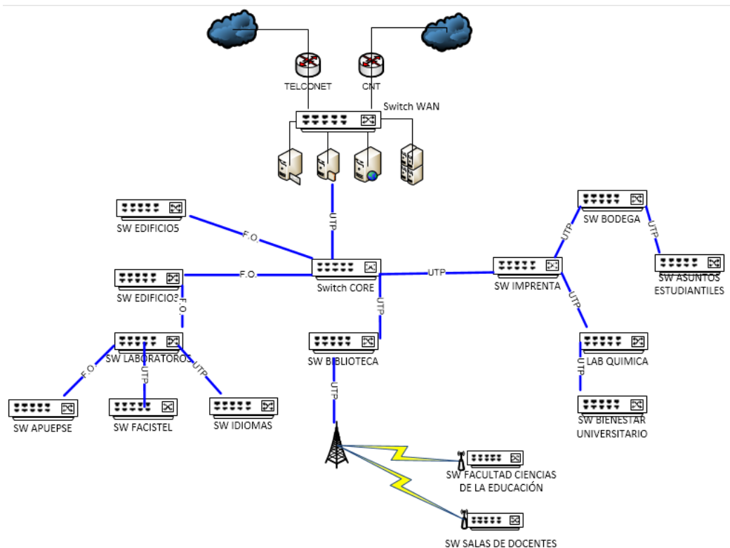
Figura 2.1 Esquema de arquitectura de red plana
