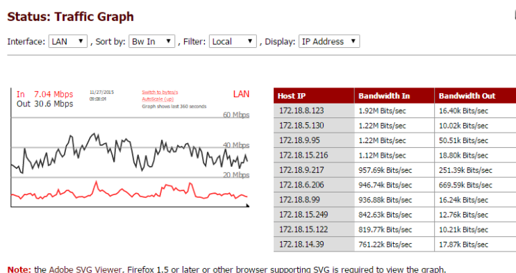
Figura 3.3 Consumo de ancho de banda por direcciones IP, red Wireless.
