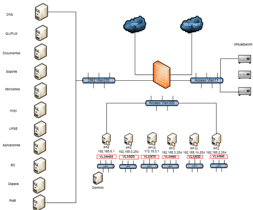
Figura 2.23. Arquitectura de Seguridad a nivel de Firewall
