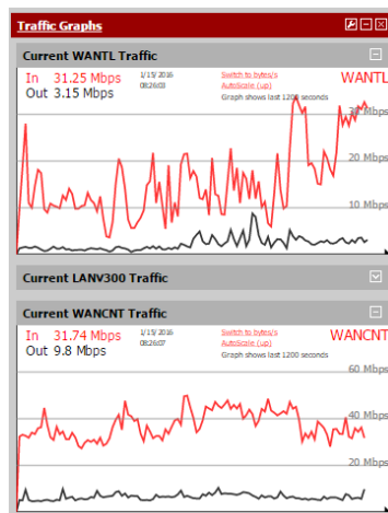
Figura 3.2 Consumo de ancho de banda por interfaces de proveedores
