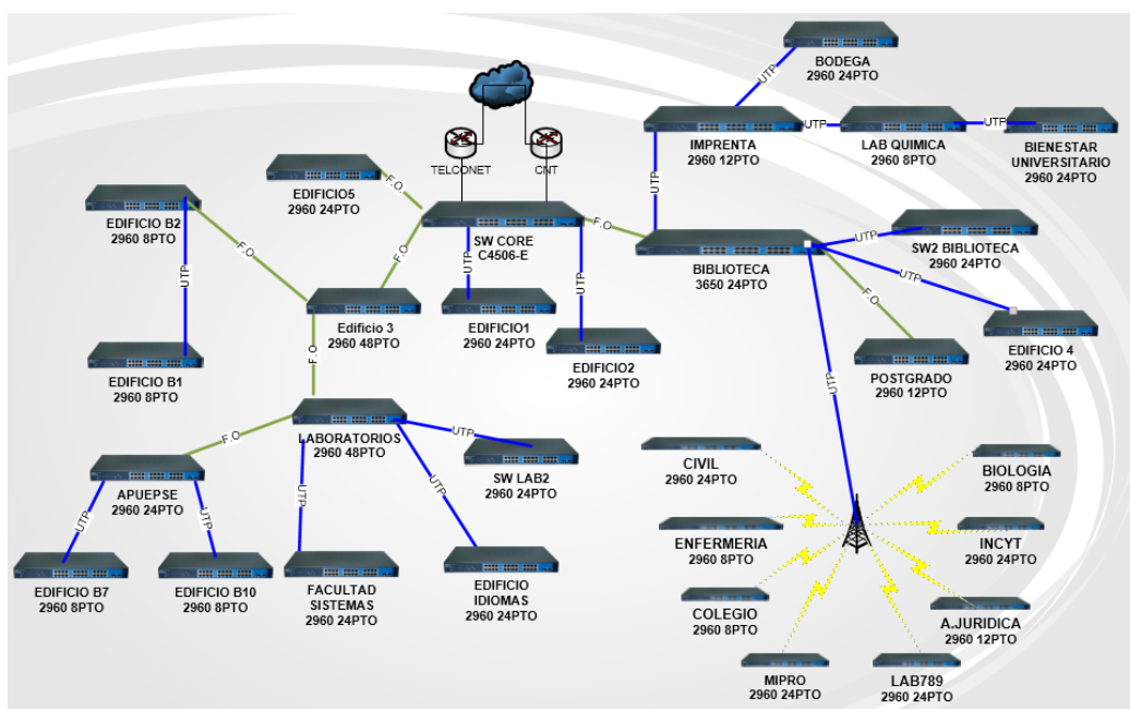
Figura 2.3 Implementación de la nueva arquitectura.
