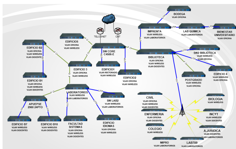
Figura 2.4 Implementación de Vlans.
