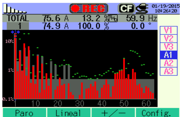
Figura 7.11 Medición en tiempo real de Armónico de Corriente A1 Panel 220 V
