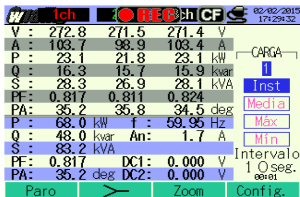
Figura 7.15 Mediciones Instantáneas de W Panel 460V
