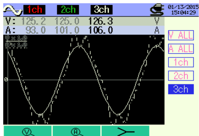
Figura 7.8 Mediciones Instantáneas de Onda Canal 3 Panel 220 V
