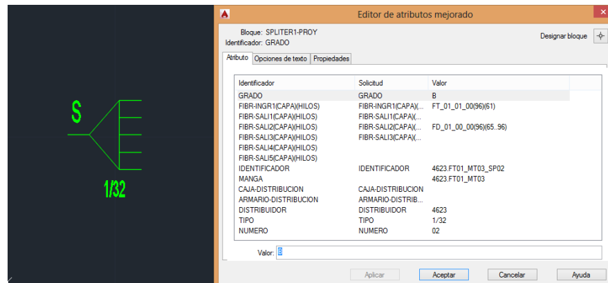
Figura 3.16 Splitter
