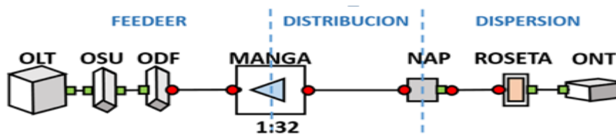
Figura 3.11 Modelo residencial
