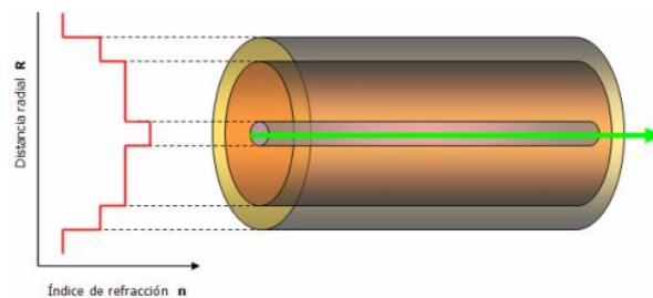
Figura 2 10 Fibra monomodo [4]
