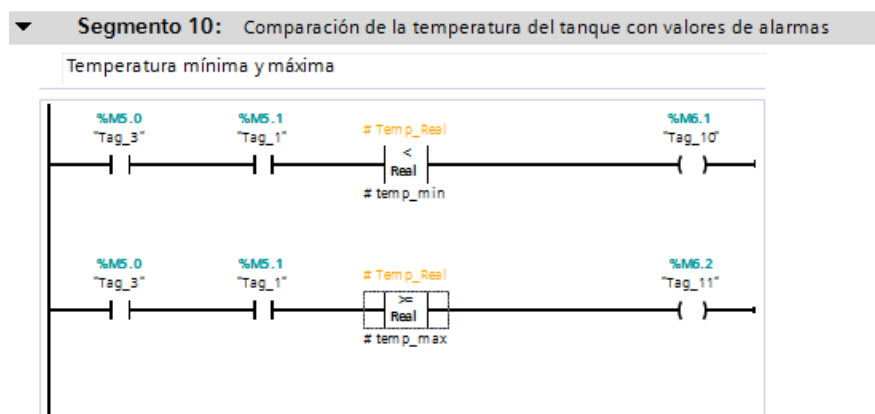
Figura 3.24 Implementación del décimo segmento en TIA PORTAL.
