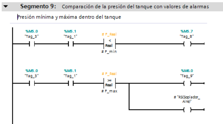
Figura 3. 23 Implementación del noveno segmento en TIA PORTAL.
