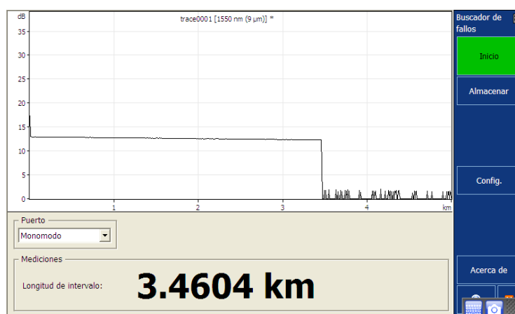
Figura C.1: OTDR Gráfico dB vs. Km FAT B4 Red GPON – FTTH Cdla. Las Garzas
