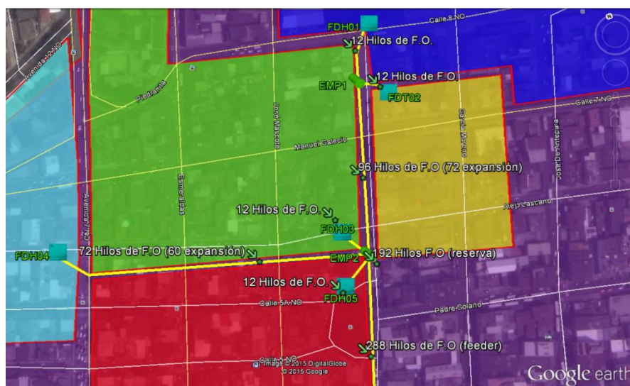
Figura 3.5: Mapa Geo-referenciado ampliado Red GPON - FTTH Ruta 13
