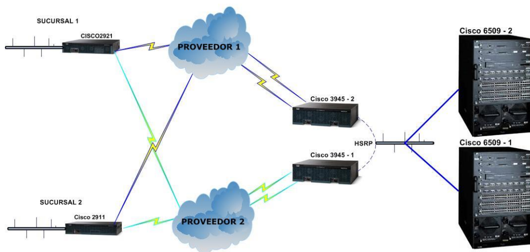
Figura 2. 2: Esquema de Conexión propuesto en Centro de Computo Principal.
