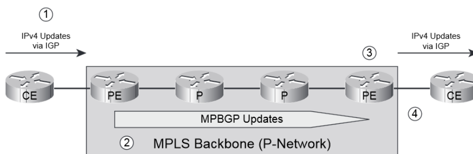
Figura 1.4: Flujo de Enrutamiento de Extremo a Extremo [2].
