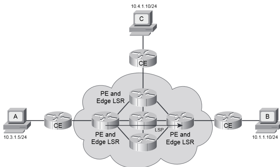
Figura 1. 2: Uso de MPLS en una Red IP [2].
