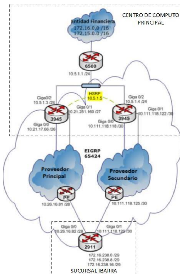
Figura 2.3: Esquema de Conexión en Instalación de Sucursal Piloto.
