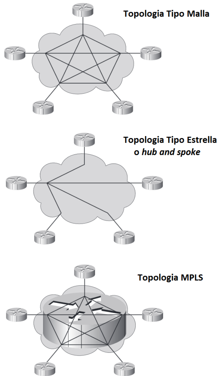
. Figura 1. 1: Topologías de Red Tradicional y MPLS [2].
