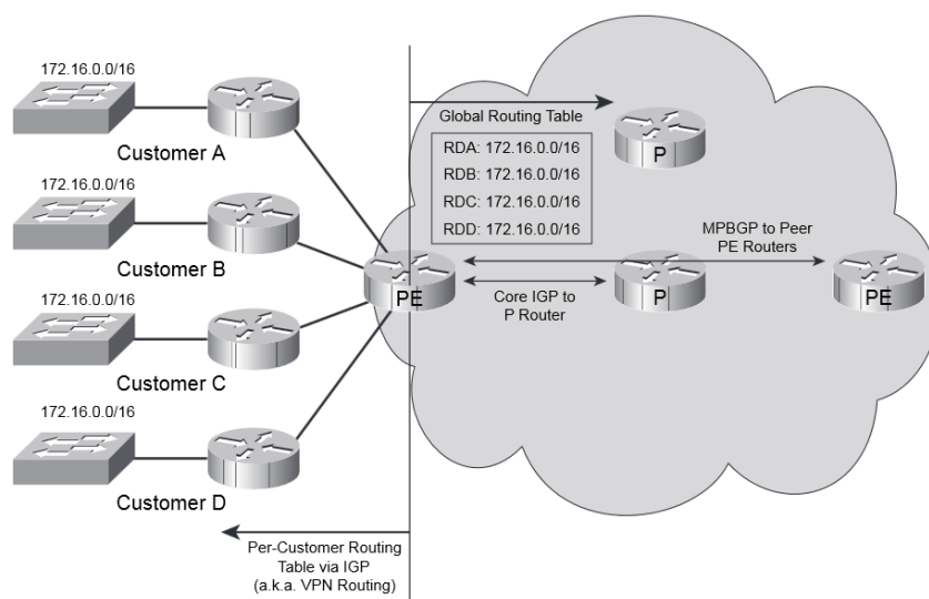
Figura 1.3: Arquitectura de Router PE [2].
