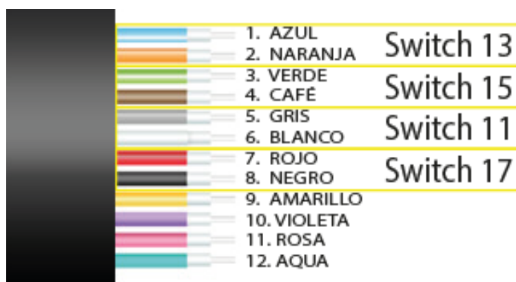
Figura 2.17 Asignación de hilos de la tercera fibra óptica multimodo que conectan el centro de cómputo con los bloques 4, 5, 6 y 7
