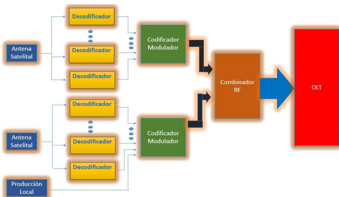
Figura 3.12: Bloques del headend digital propuesto [19].
