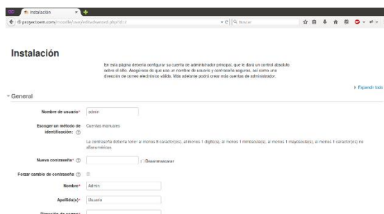
Figura 2.20 Pagina inicial de configuración de Moodle.
