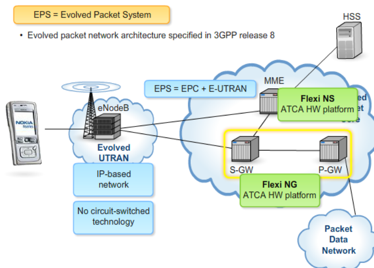
Figura 1.2: Arquitectura de red LTE [1]
