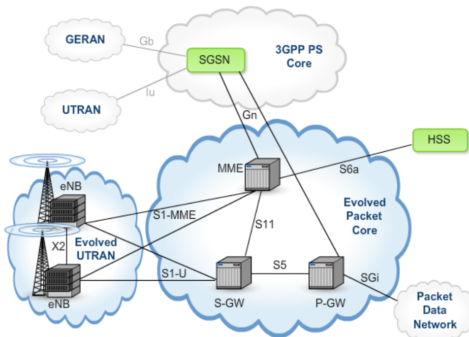
Figura 1.3: Interfaces de red LTE
