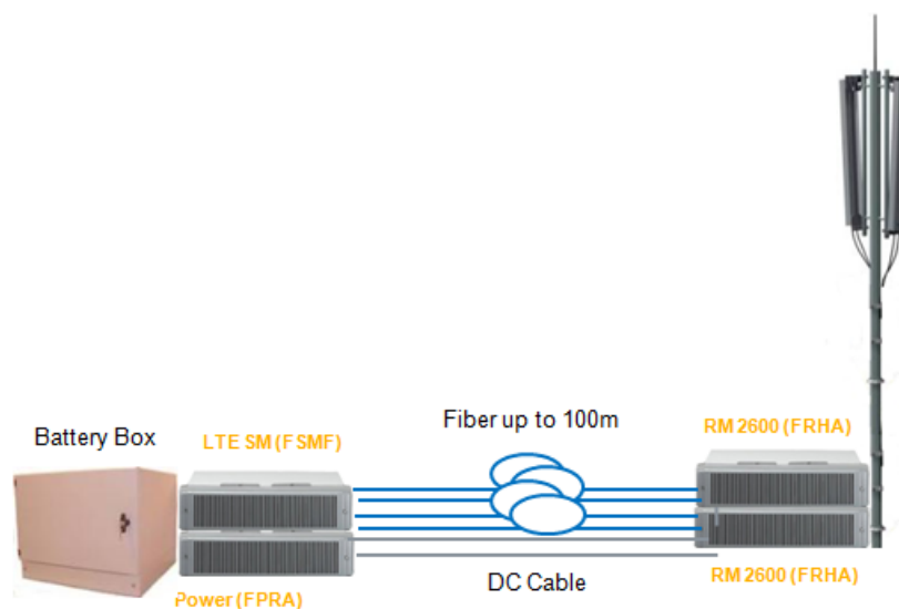
Figura 2.3: Solución eNodeB Flexi Multiradio concentrada [6]
