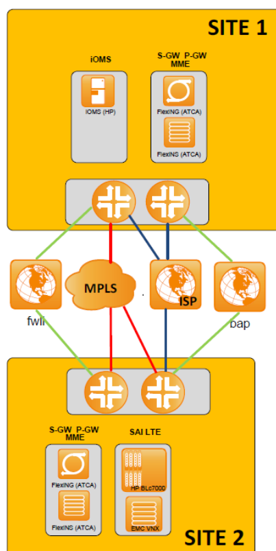
Figura 2.2: Diseño de alto nivel de EPC LTE [5]
