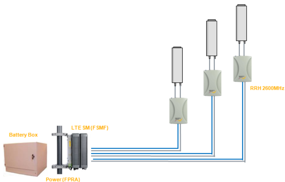
Figura 2.4: Solución eNodeB Flexi Multiradio distribuida [6]
