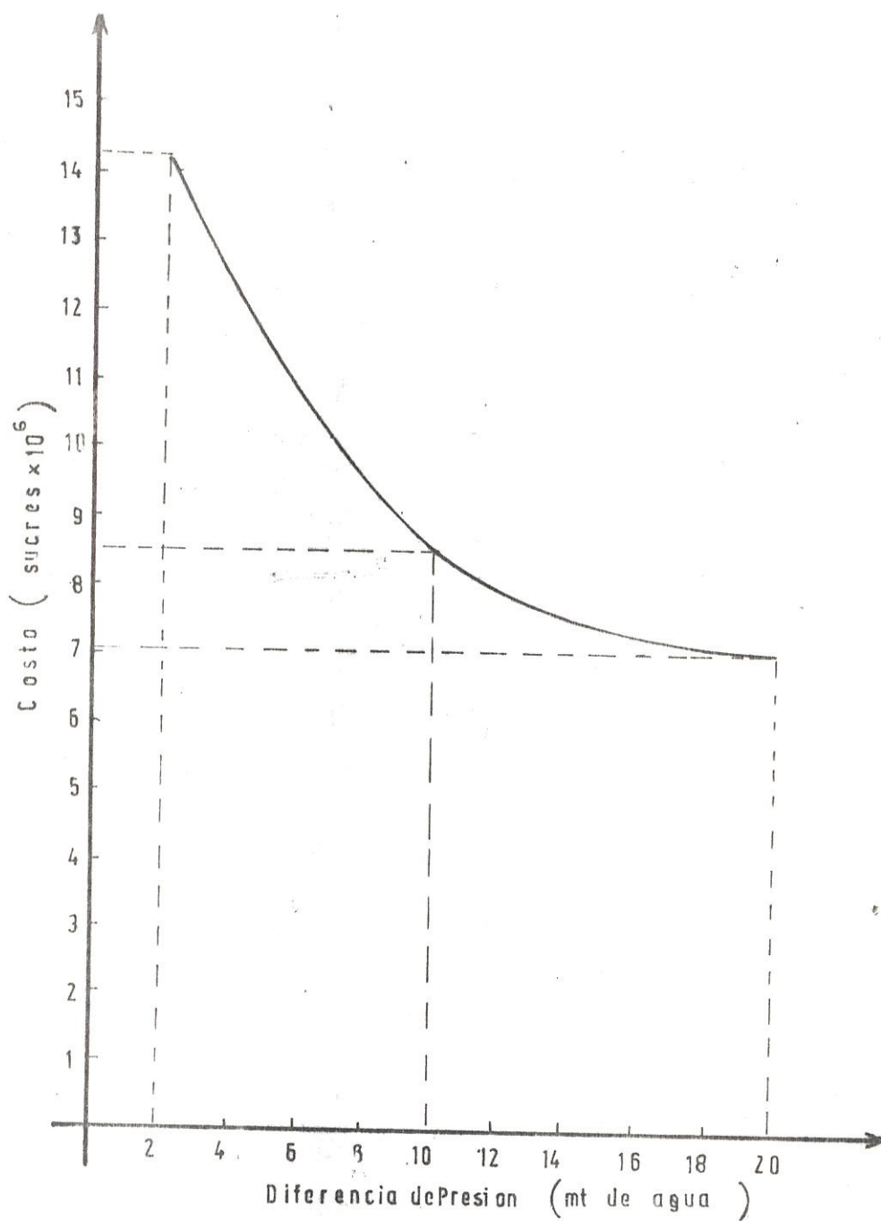
GRAFICA DE LA VARIACION DEL COSTO DE LA RED CON LAS DIFERENCIAS DE PRESIONES.
