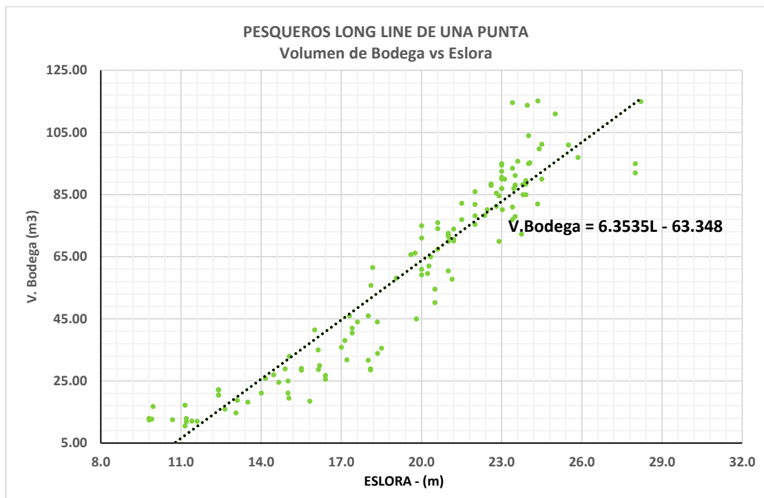
Figura B.2.18.- Tendencia de V. Bodega vs L
