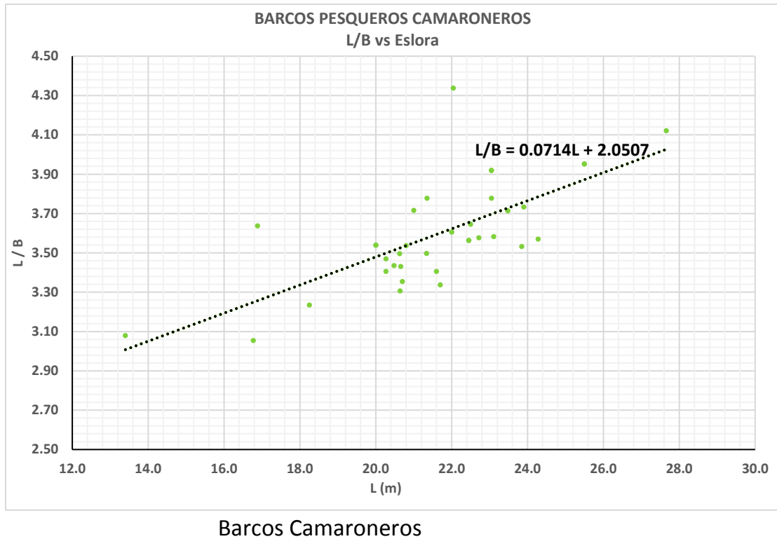
Figura B.2.1.- Tendencia de L/B vs L
