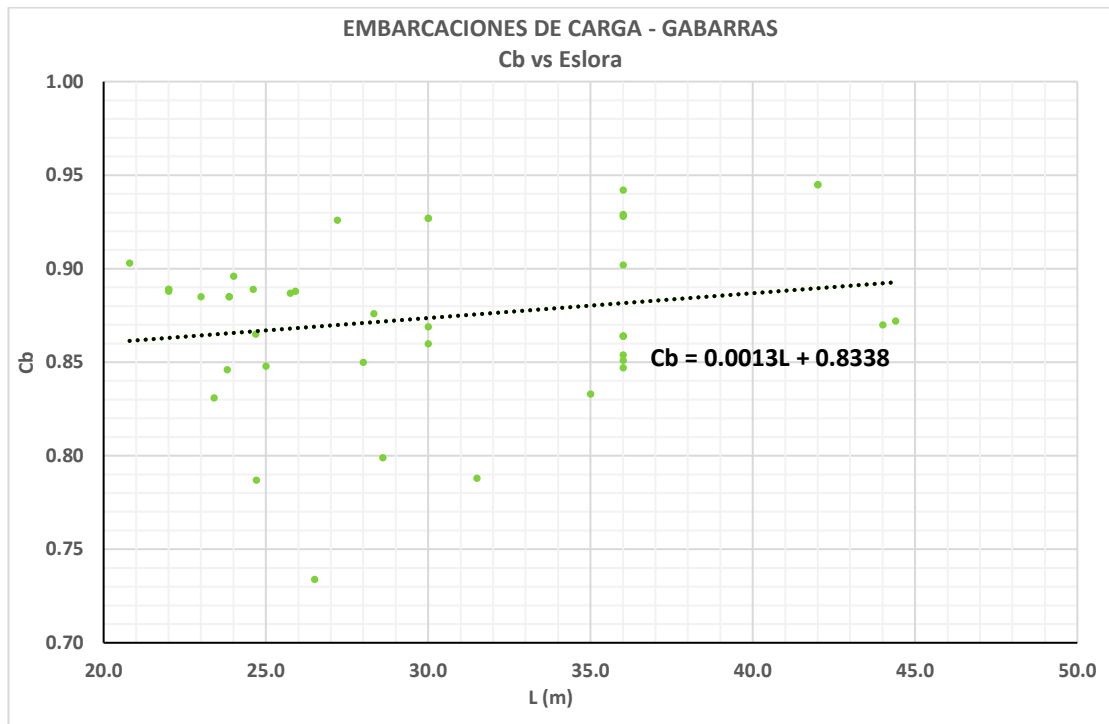
Figura B.3.4.- Tendencia de C_b vs L
