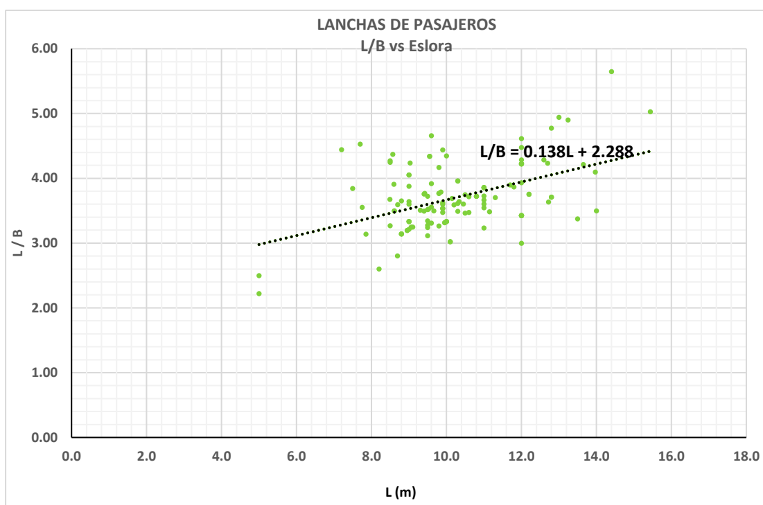
Figura B.1.1- Tendencia de L/B vs L
