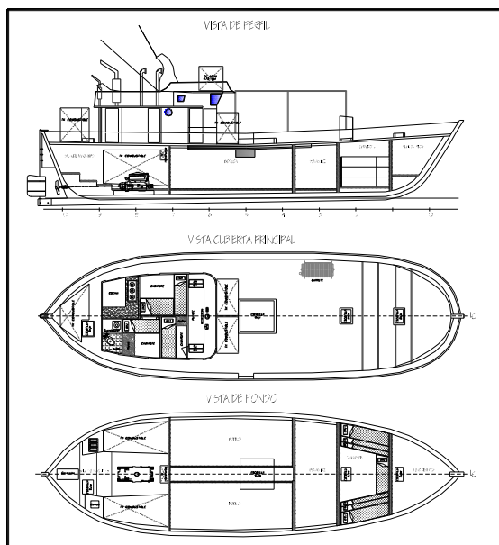
Figura 5.10.- Plano Barco Pesquero Long Line dos puntas #50 – [Tabla A.2.16] - [Anexo A] - Manta
