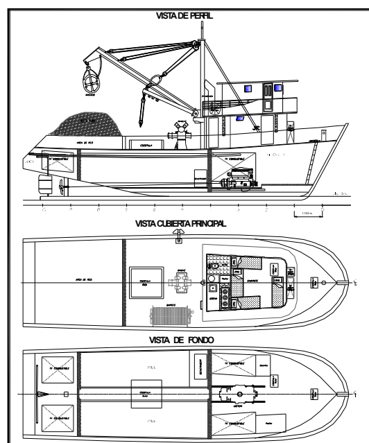
Figura 5.6.- Plano Barco Cerquero #27 – [TablaA.2.4] - [Anexo A] - Manta
