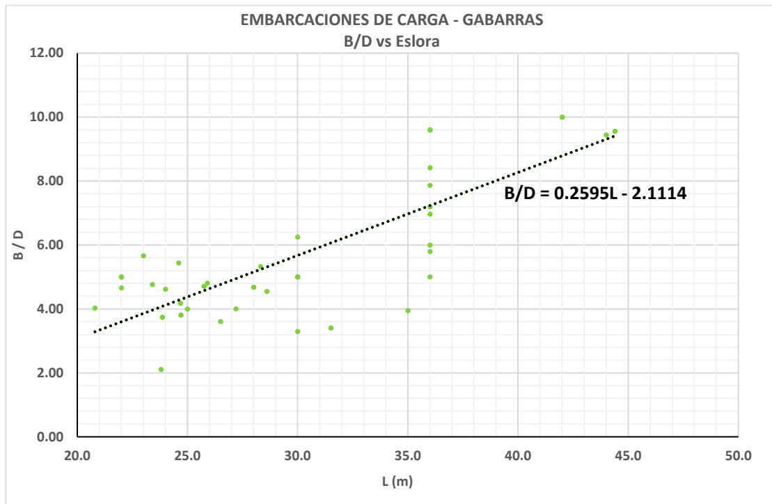
Figura B.3.2.- Tendencia de B / D vs L
