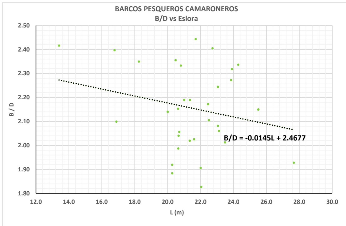
Figura B.2.2.- Tendencia de B / D vs L
