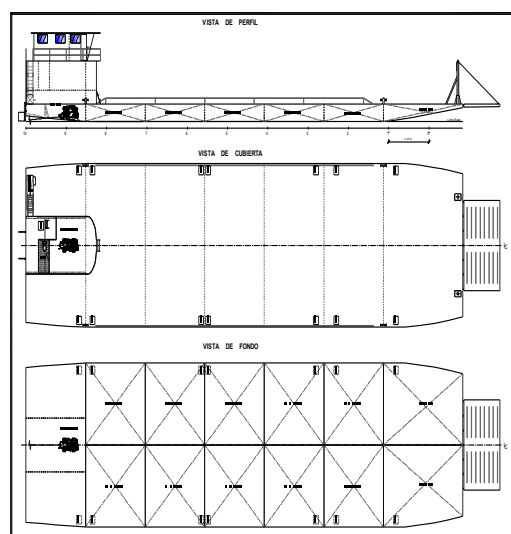
Figura 5.14.- Plano GABARRA #2 – [Tabla A.3.3] - [Anexo A] El Coca
