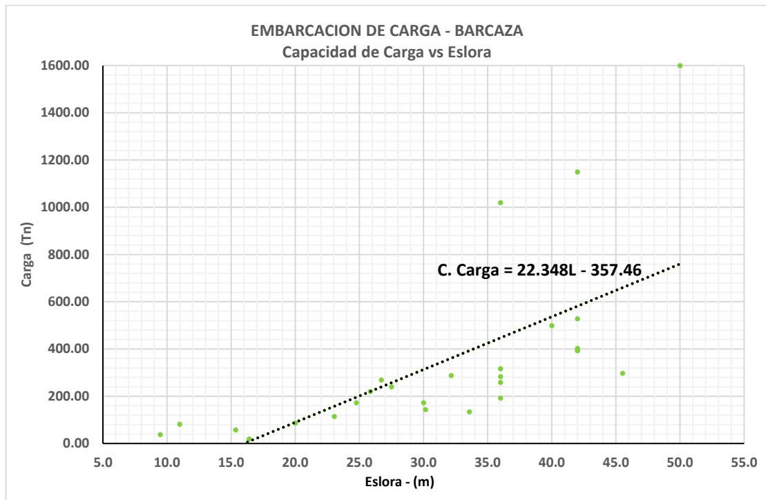
Figura B.3.12.- Tendencia de Capacidad de Carga vs L
