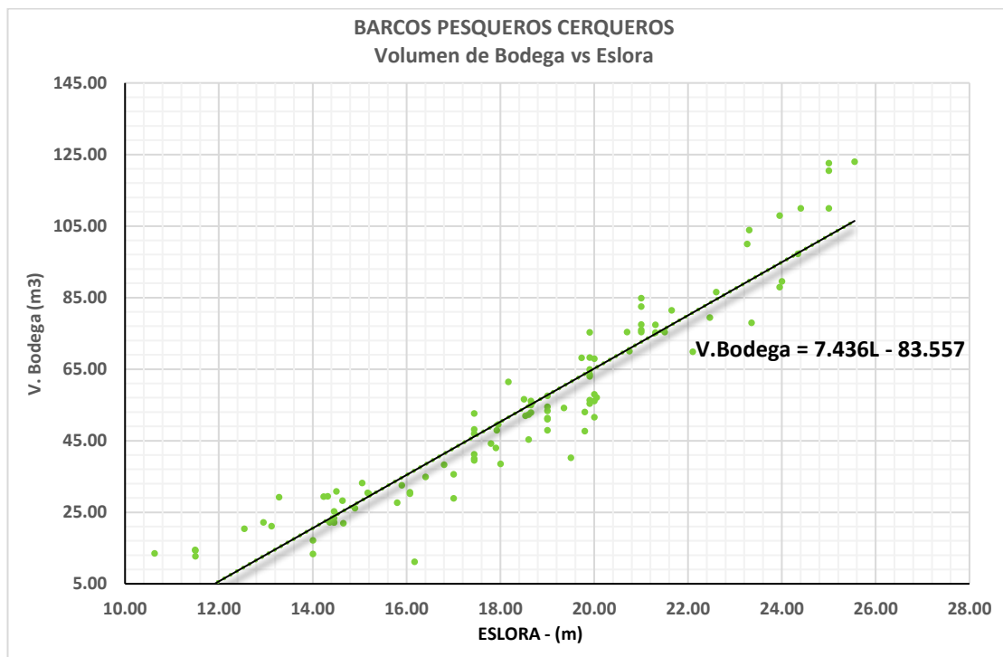
Figura B.2.12.- Tendencia de Volumen de Bodega vs L
