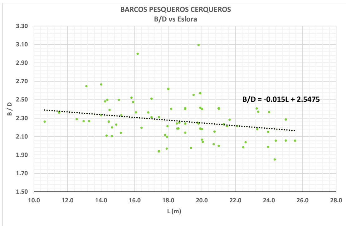
Figura B.2.8.- Tendencia de B / D vs L
