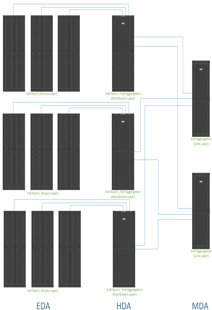
Figura 3.20: Topología a Implementar en el CPD [24].
