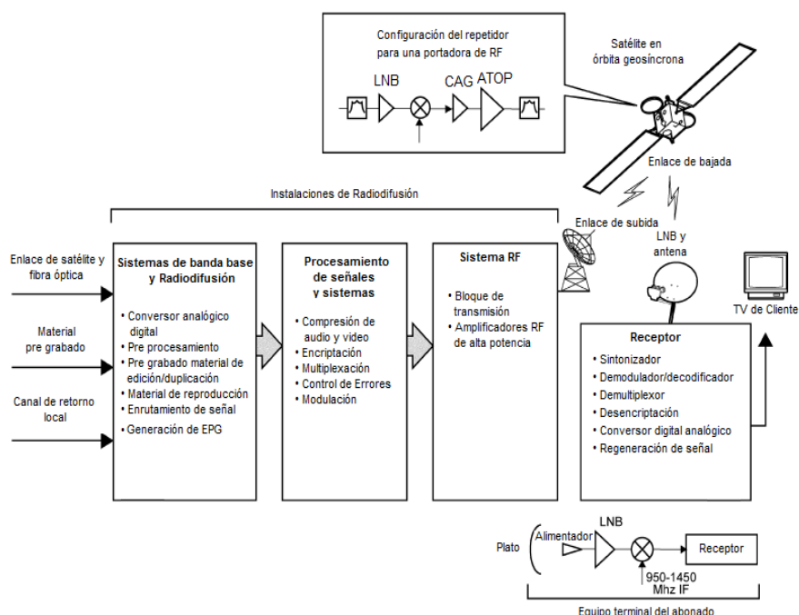
Figura 2.1 Estructura del modelo DTH [8]
