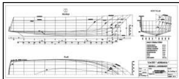
Figura 3. Planos de líneas de formas.
