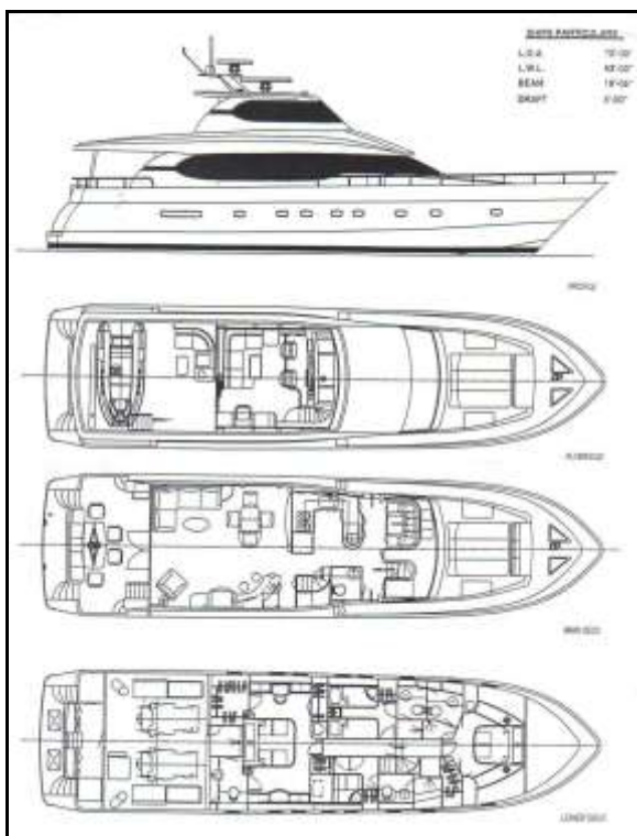
Figura 2. Planos de yate del catálogo.
