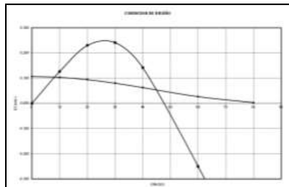
Figura 6. Gráfico de GZ y GZe.
