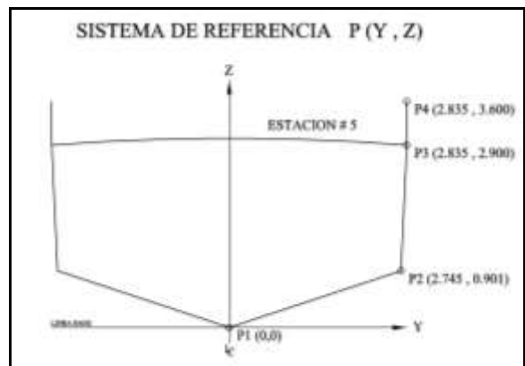
Figura 7. Sistema de referencia de puntos. Fuente: propia
