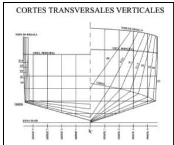
Figura 8. Cortes transversales verticales. Fuente: propia
