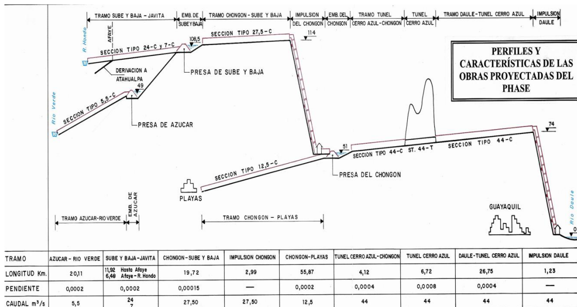
Gráfico 8: Esquema y características de las obras proyectadas en el PHASE
