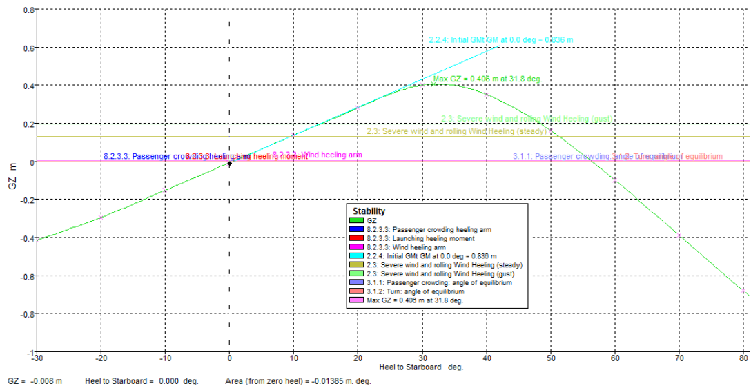
Figura No. 28. Curva de estabilidad a grandes ángulos – Condición I. Fuente: Hydromax – Versión de prueba.
