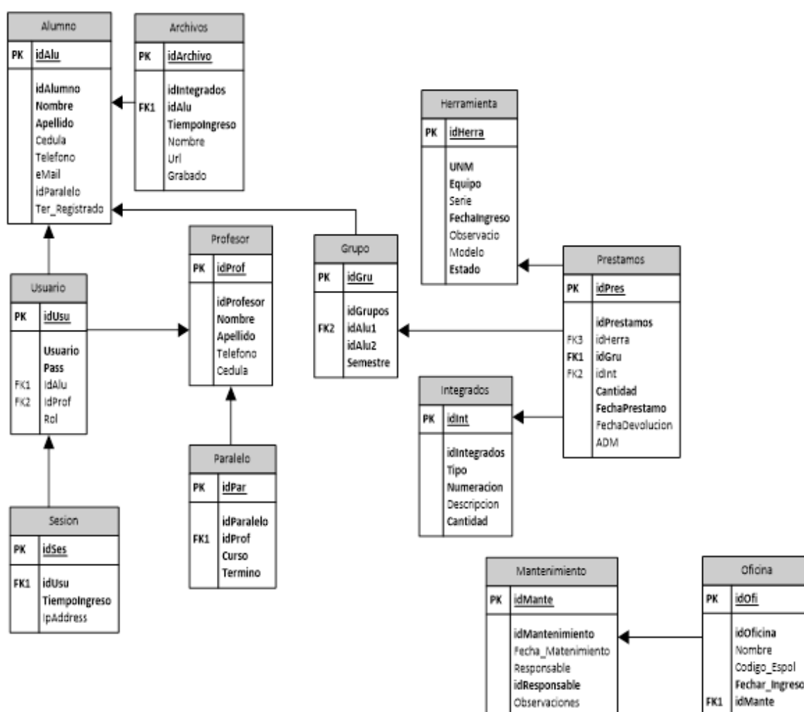
Figura 2.2 Modelo Lógico
