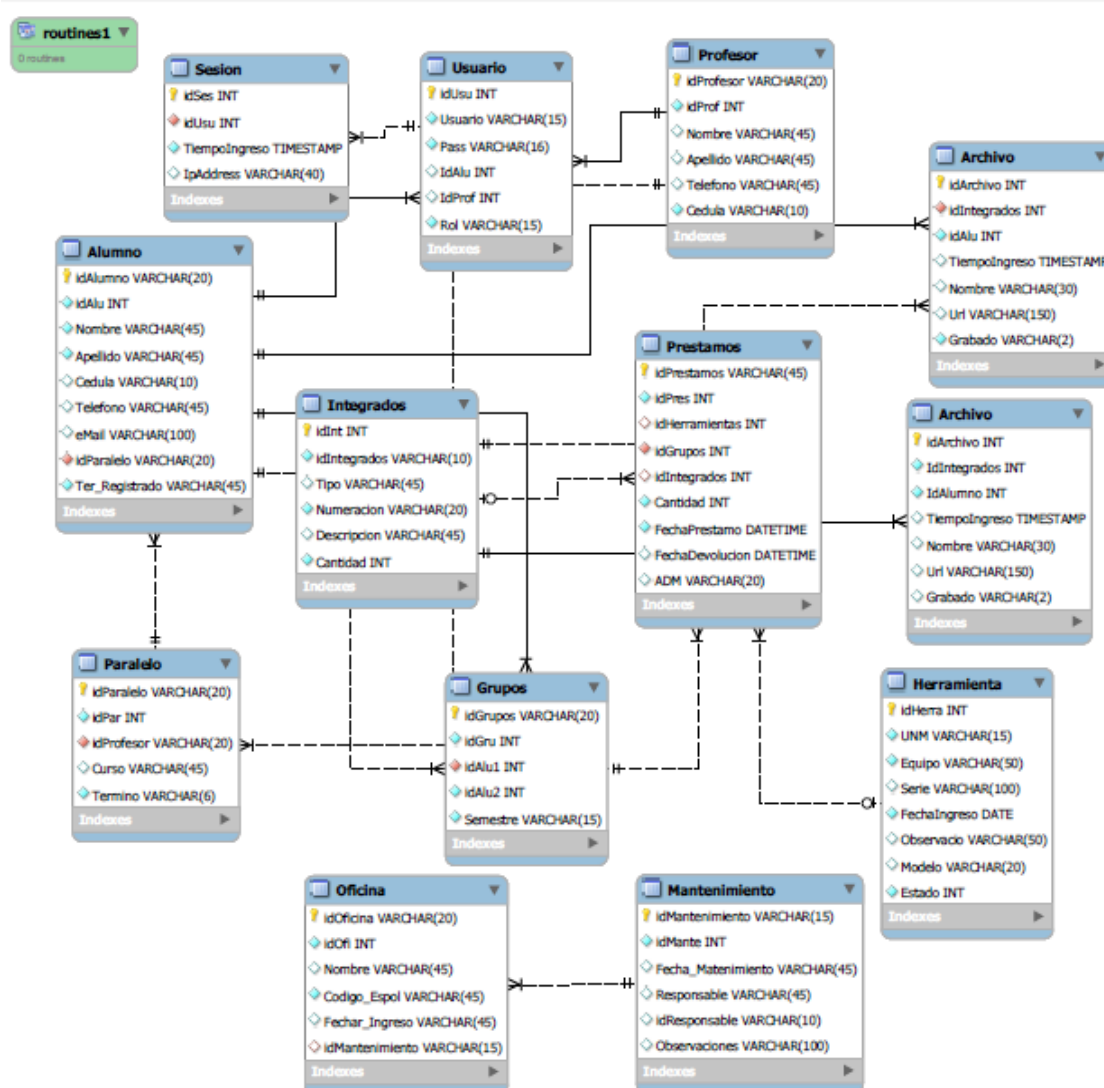
Figura 2.3. Modelo Lógico Normalizado
