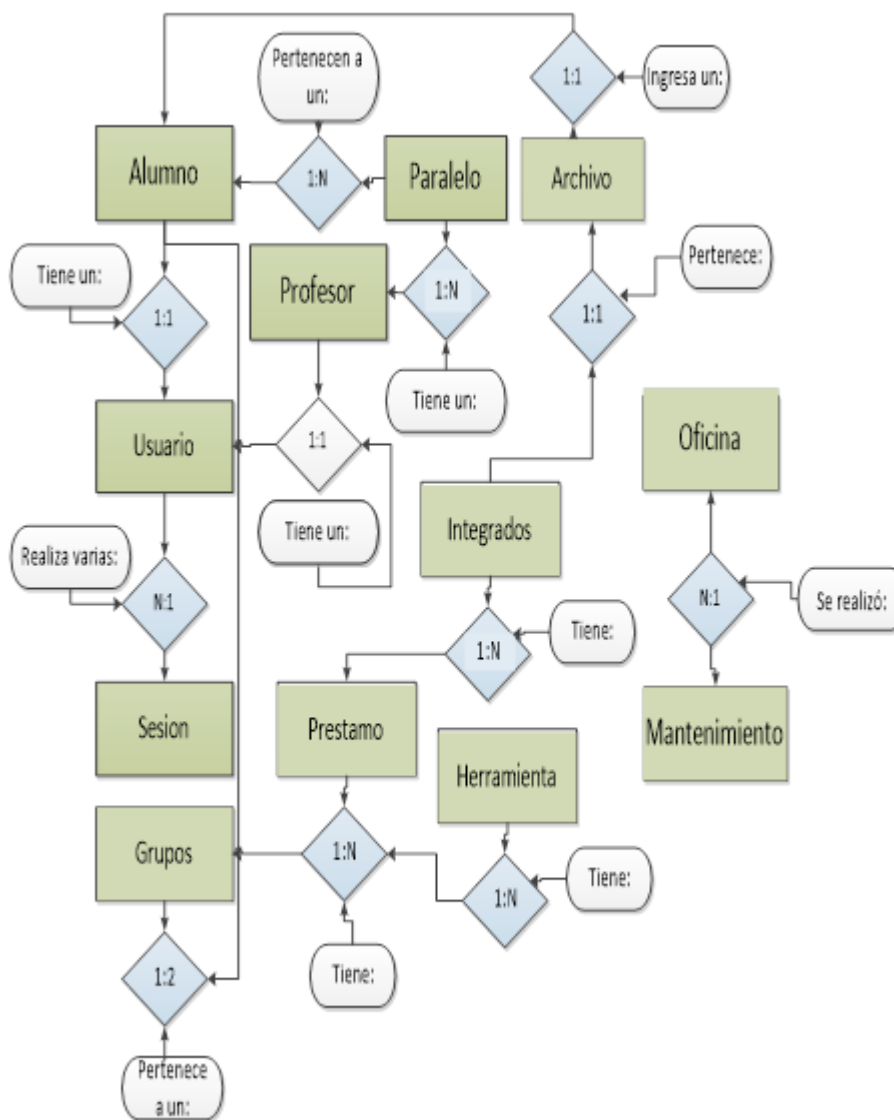
Figura 2.1 Modelo Conceptual
