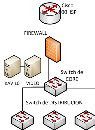
Figura 1.2 Topología de seguridad
