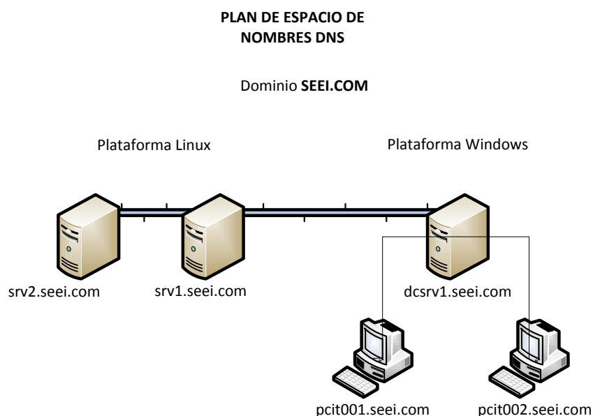
Figura 2.4 Plan de espacios de nombres DNS
