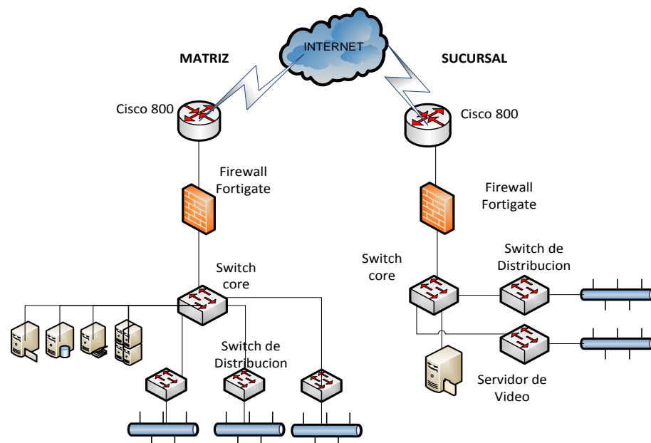
Figura 1.1 Diagrama de la Infraestructura TI
