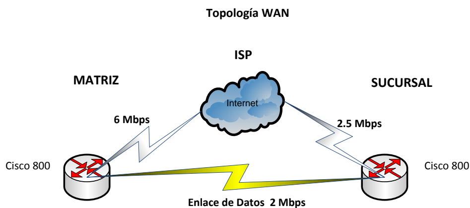
Figura 1.3 Análisis de la Topología WAN
