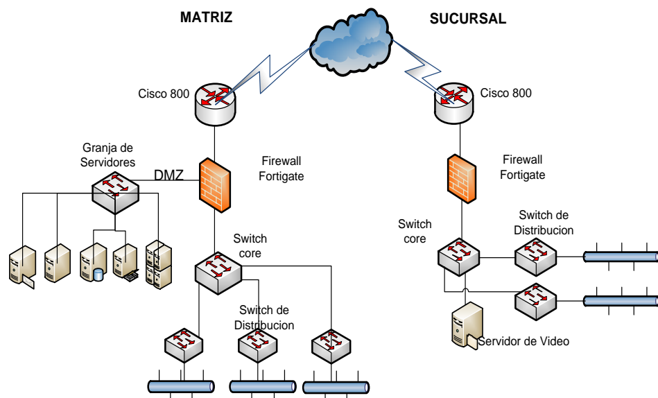
Figura 2.1 Diseño de la infraestructura TI
