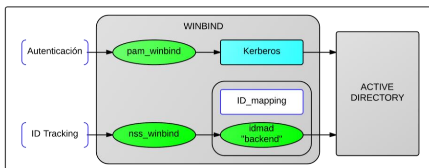
Figura 3.1 Funcionamiento de Winbind
