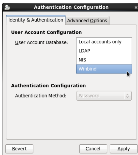
Figura 3.20 Herramienta de autenticación tab 1
