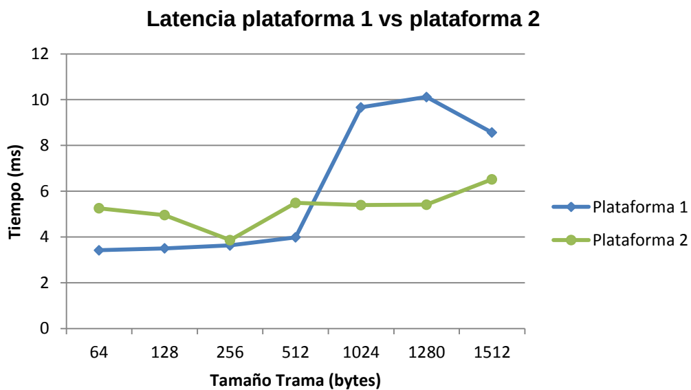
Figura 4.4 Comparativa de latencias entre plataformas
