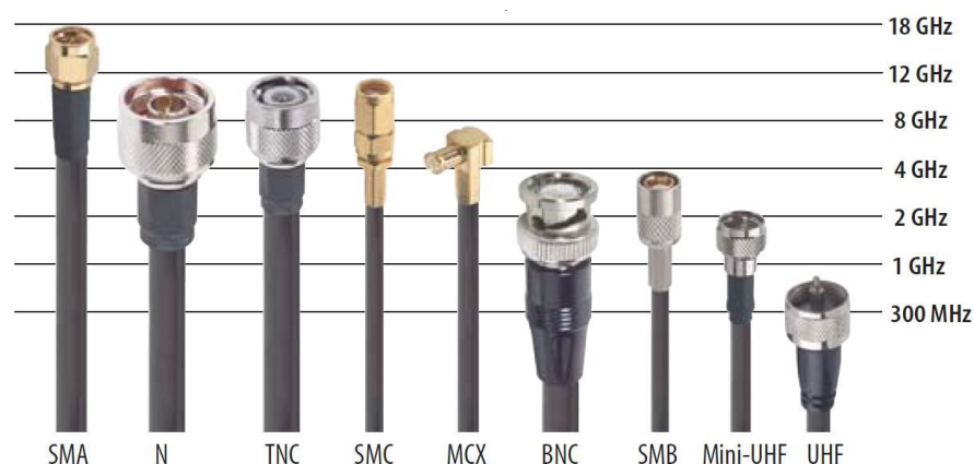
Figura 2.15 Tipo de cables coaxiales [9]
