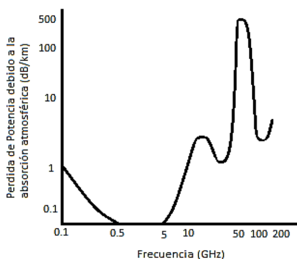
Figura 2.7 Propagación de microondas en la atmosfera [5]
