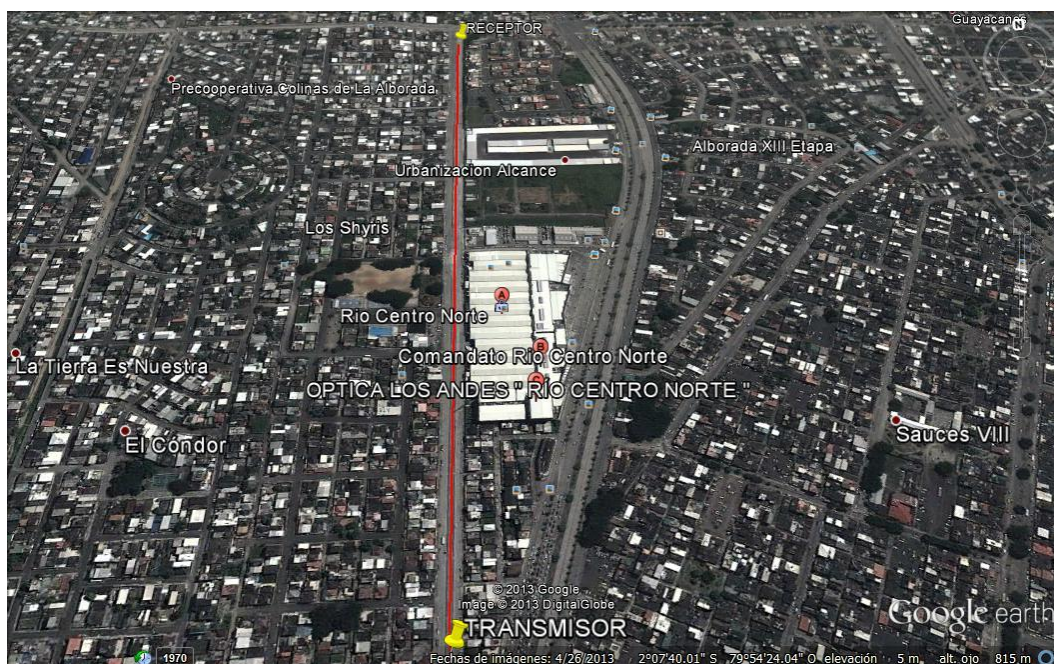
Figura 3.2 Radioenlace Alborada
