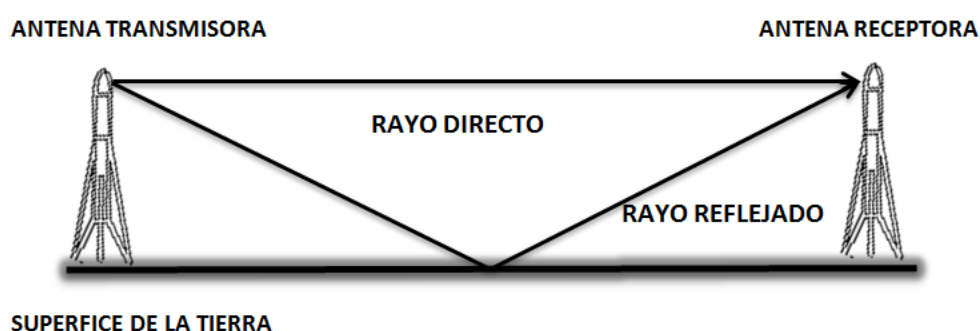
Figura 2.21 Modelo de Tierra Plana
