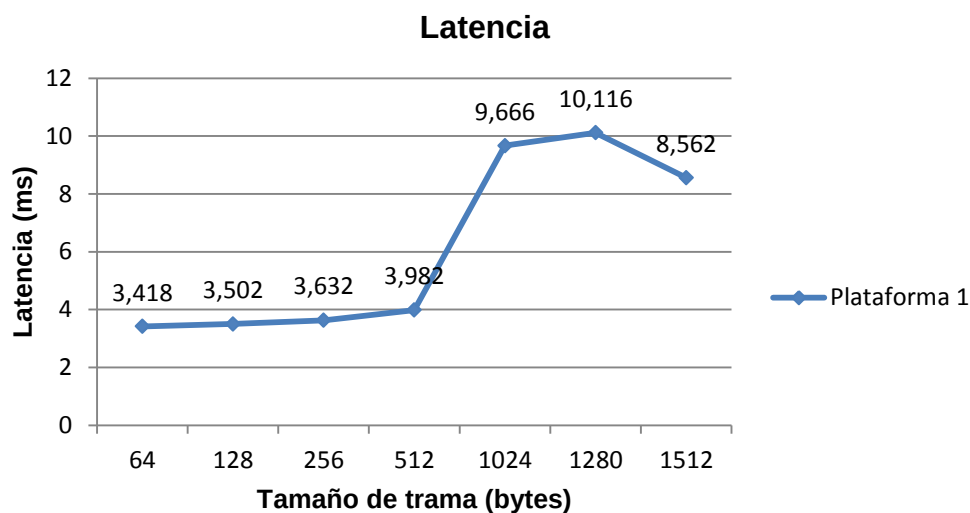
Figura 4.2 Latencia de la plataforma 1
