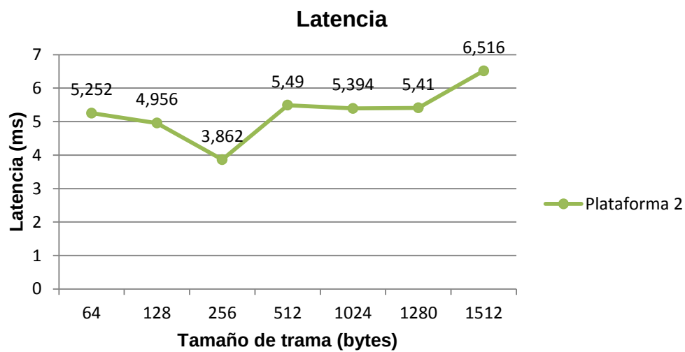
Figura 4.3 Latencia de la plataforma 2
