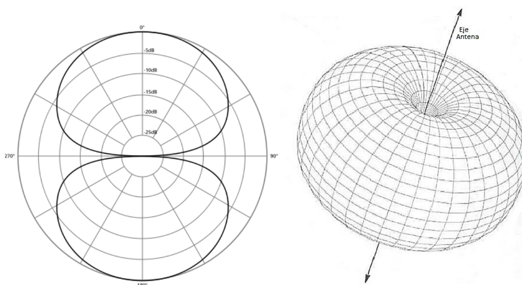
Figura 2.8 Patrón de radiación de una antena omnidireccional
