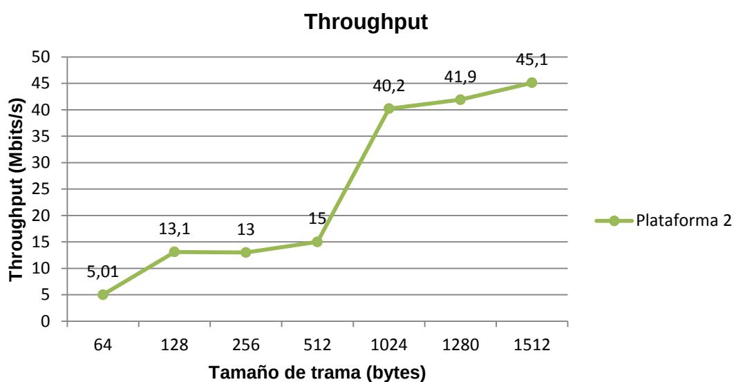
Figura 4.6 Throughput plataforma 2
