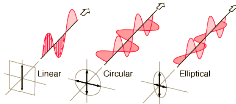
Figura 2.5 Tipos de polarización [4]
