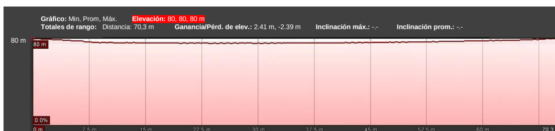
Figura 3.3 Perfil radioenlace EDCOM
