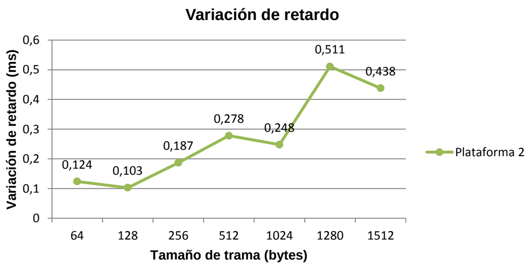
Figura 4.6 Variación de retardo plataforma 2
