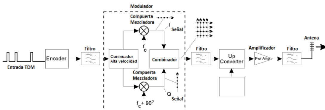
Figura 2.12 Diagrama de bloques del transmisor [6]
