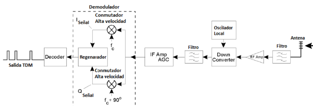
Figura 2.13 Diagrama de bloques del receptor [7]
