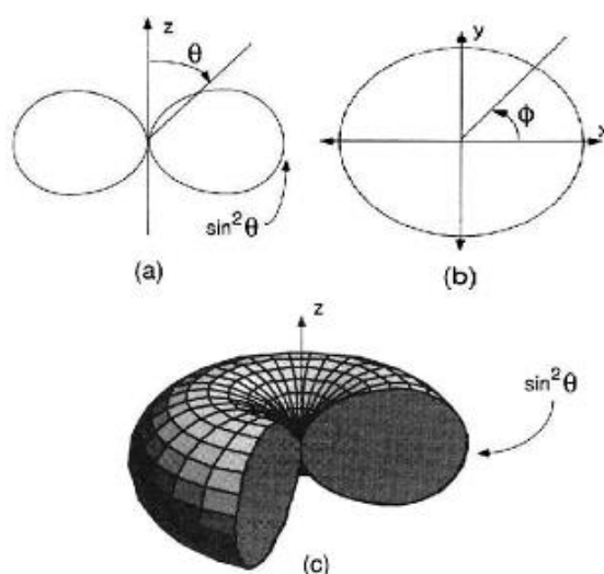
Figura 2.2 Patrones de radiación a) Patrón de elevación b) Patrón de azimuth c) Patrón de radiación 3D [2]
