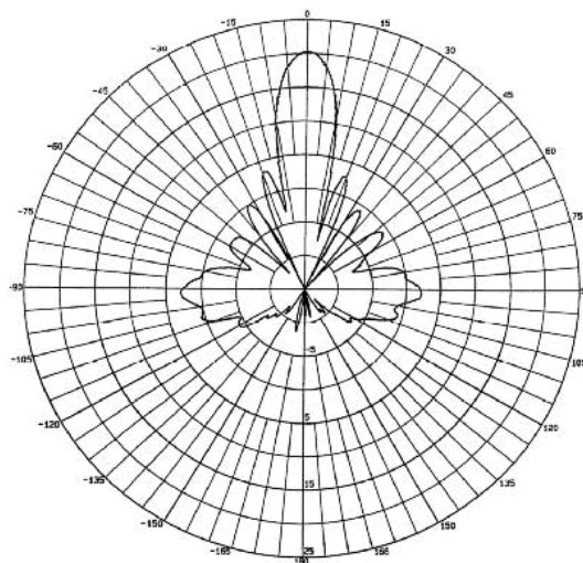
Figura 2.11 Patrón de elevación antena parabólica
