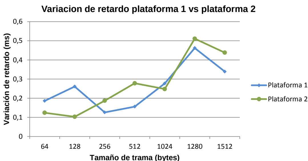
Figura 4.4 Comparativa de variación de retardo entre plataformas
