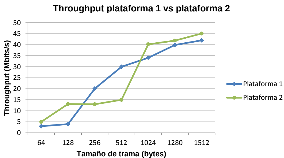
Figura 4.7 Comparativa de throughput entre plataformas
