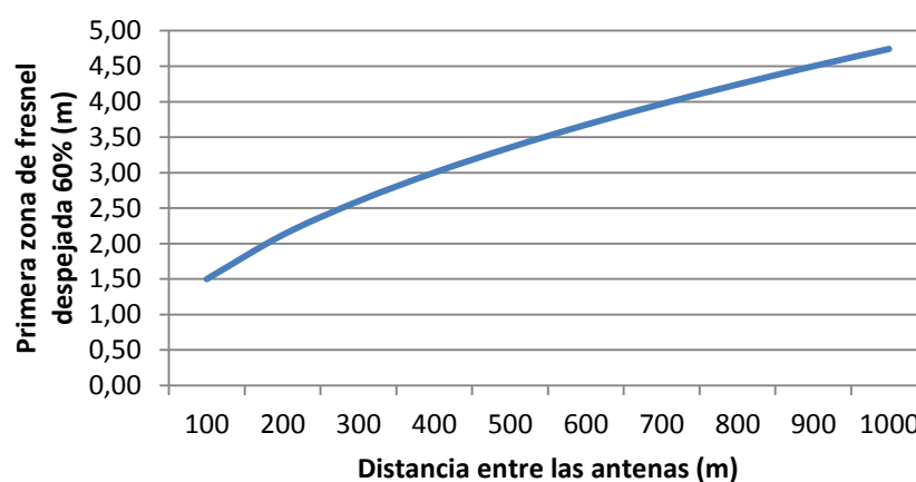
Figura 3.5 Primera zona de Fresnel despejada 60%
