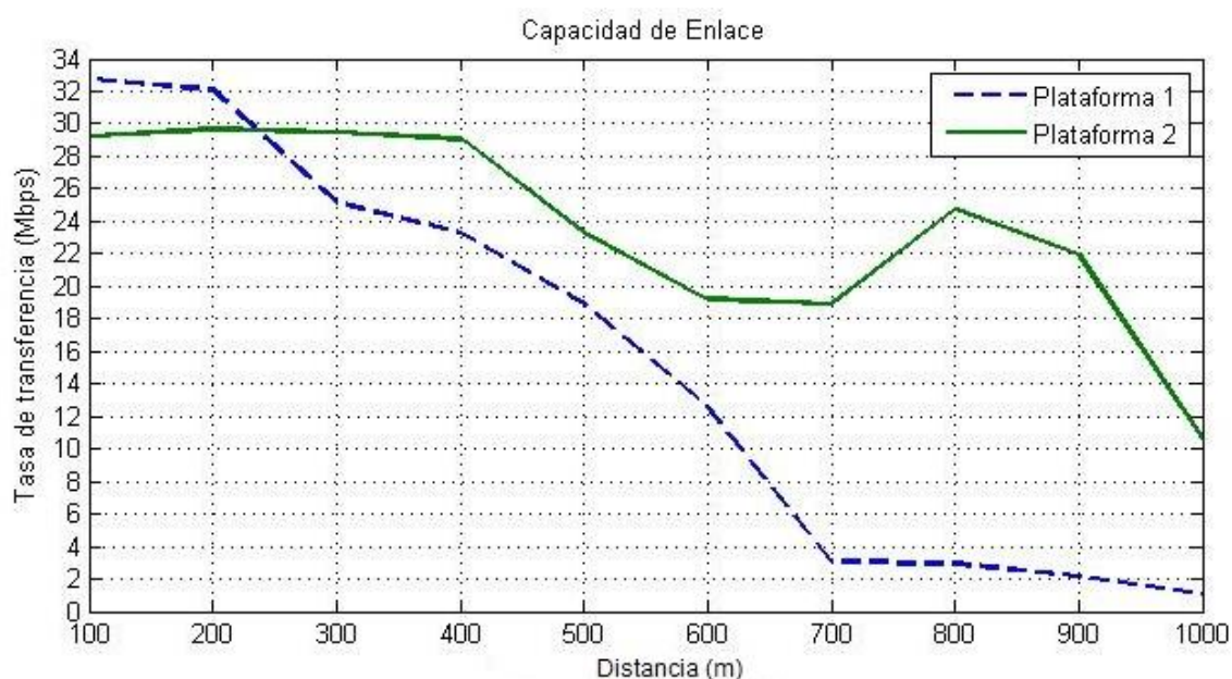
Figura 4.1 Capacidad de enlace en el sector de la Alborada
