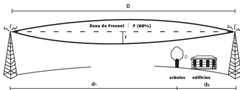
Figura 2.16 Zona de Fresnel
