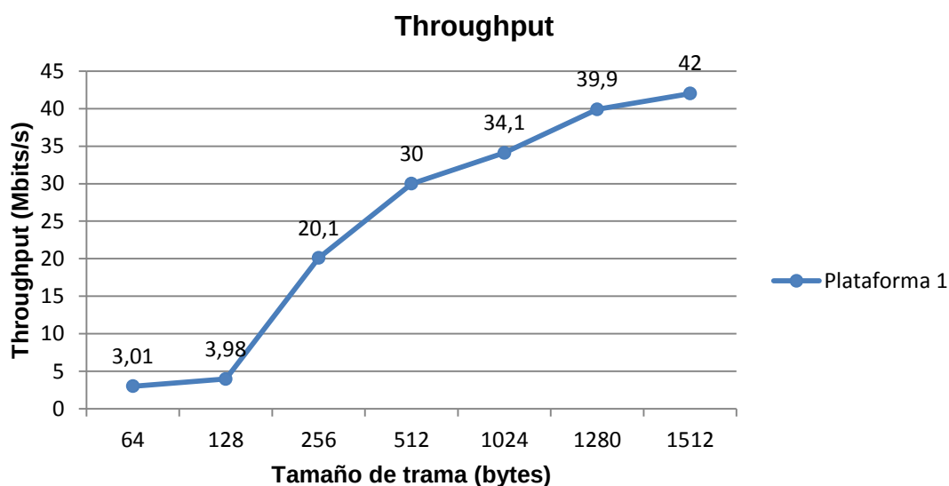
Figura 4.5 Throughput plataforma 1
