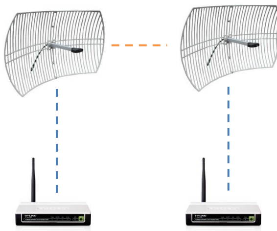
Figura 3.9 Enlace con antena rejilla (Plataforma 2)
