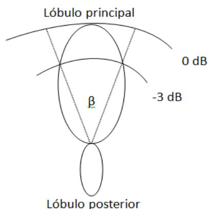
Figura 2.4 Ancho de haz de una antena
