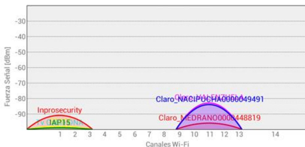
Figura 3.7 Análisis espectro en la Alborada
