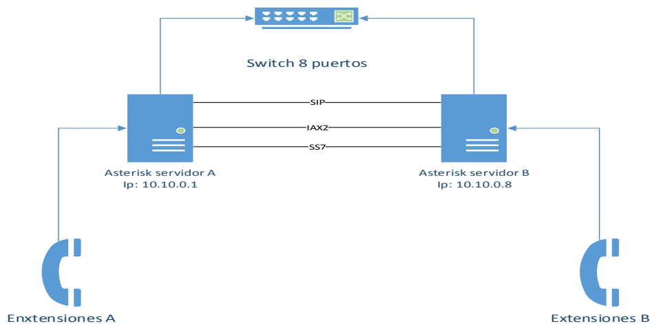
Fig. 3.2. Diagrama esquemático de conexión
