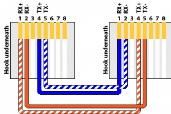
Fig. 3.1 Cable cruzado para E1/T[22]
