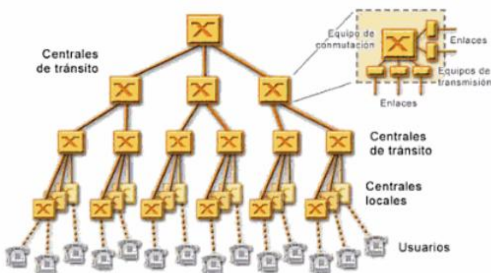
Fig.1.1. Diseño de una central telefónica convencional [1]
