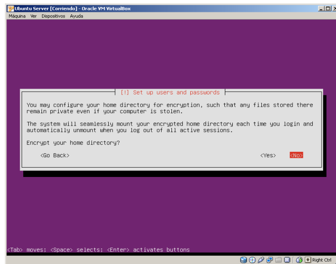
Fig.5.5 Encriptación Directorio
