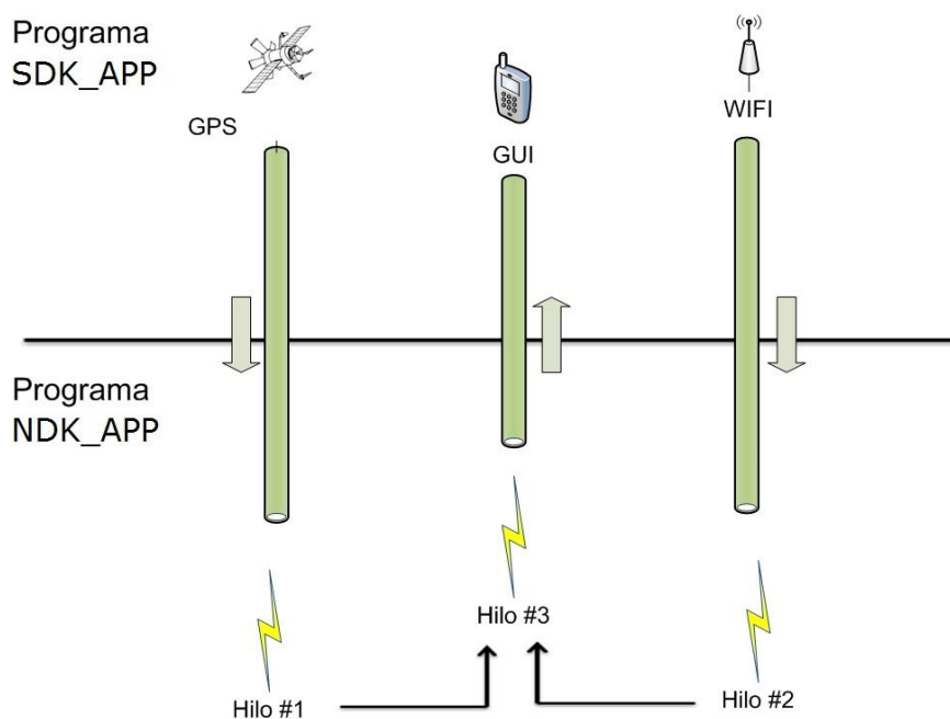
Figura 3.2. Funcionamiento de los hilos creados.
