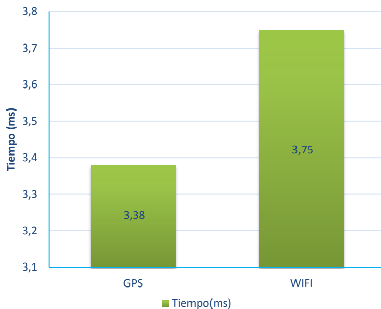
Figura 4.5. Tiempo promedio de enviar datos vía sockets entre servidor (SDK) y cliente (NDK).
