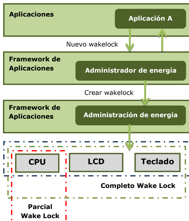
Figura 2.4. Arquitectura del administrador de energía de Android con wakelocks [9].
