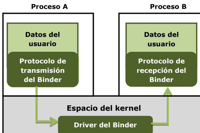
Figura 2.3. Configuración del controlador del Binder.
