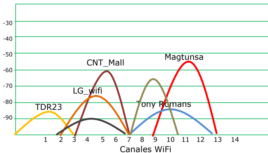
Figura 4.8. Potencia señal vs canales de WiFi
