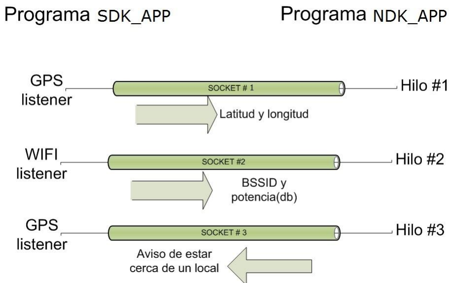
Figura 3.1. Funcionamiento de Sockets entre Programas en Java y C
