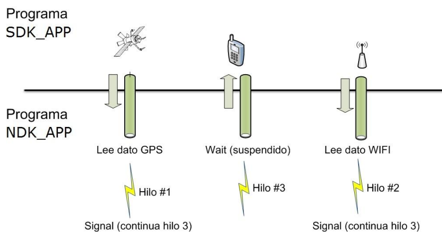
Figura 3.3. Funcionamiento Semáforos
