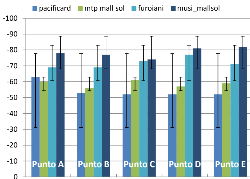
Figura 4.7. Niveles de potencia obtenidos y barras de error de una de las tiendas.
