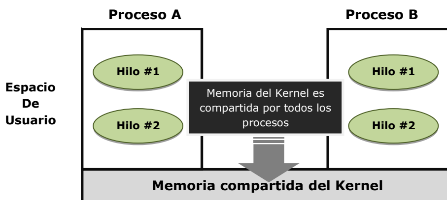
Figura 2.2. El espacio del núcleo compartido por todos los procesos.
