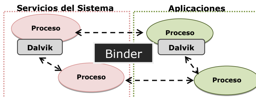
Figura 2.1. Binder, Comunicación entre Procesos.
