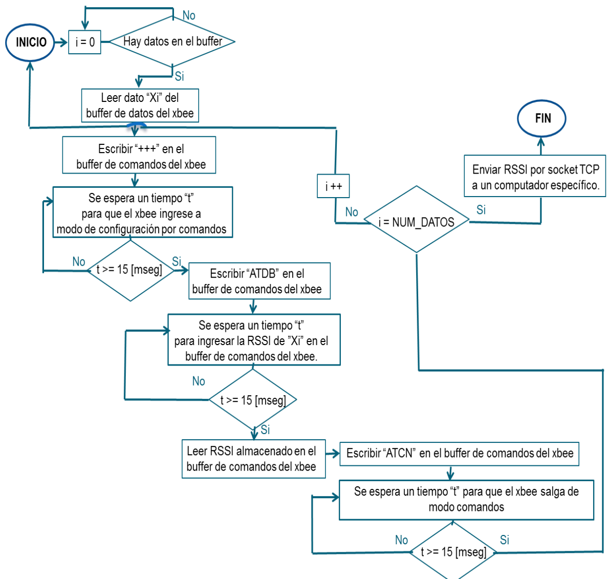
Figura 3.11 Diagrama de flujo del programa receptor
