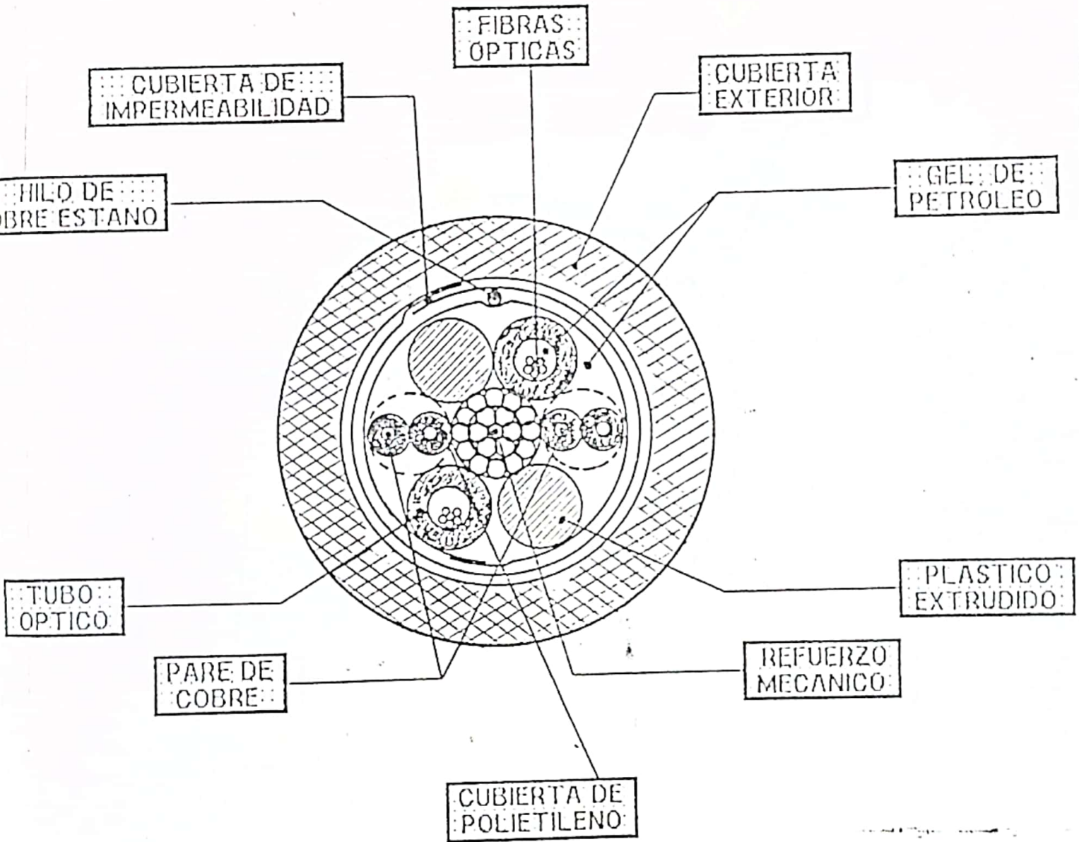
Fig. 10.1 CABLE DE FIBRA OPTICA UTILIZADO POR ALCATEL
