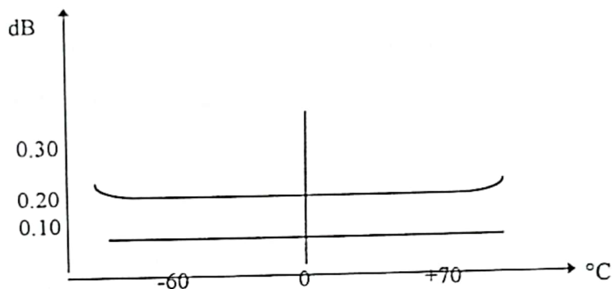
Fig. 10.5 Atenuación del empalme en función de la temperatura
