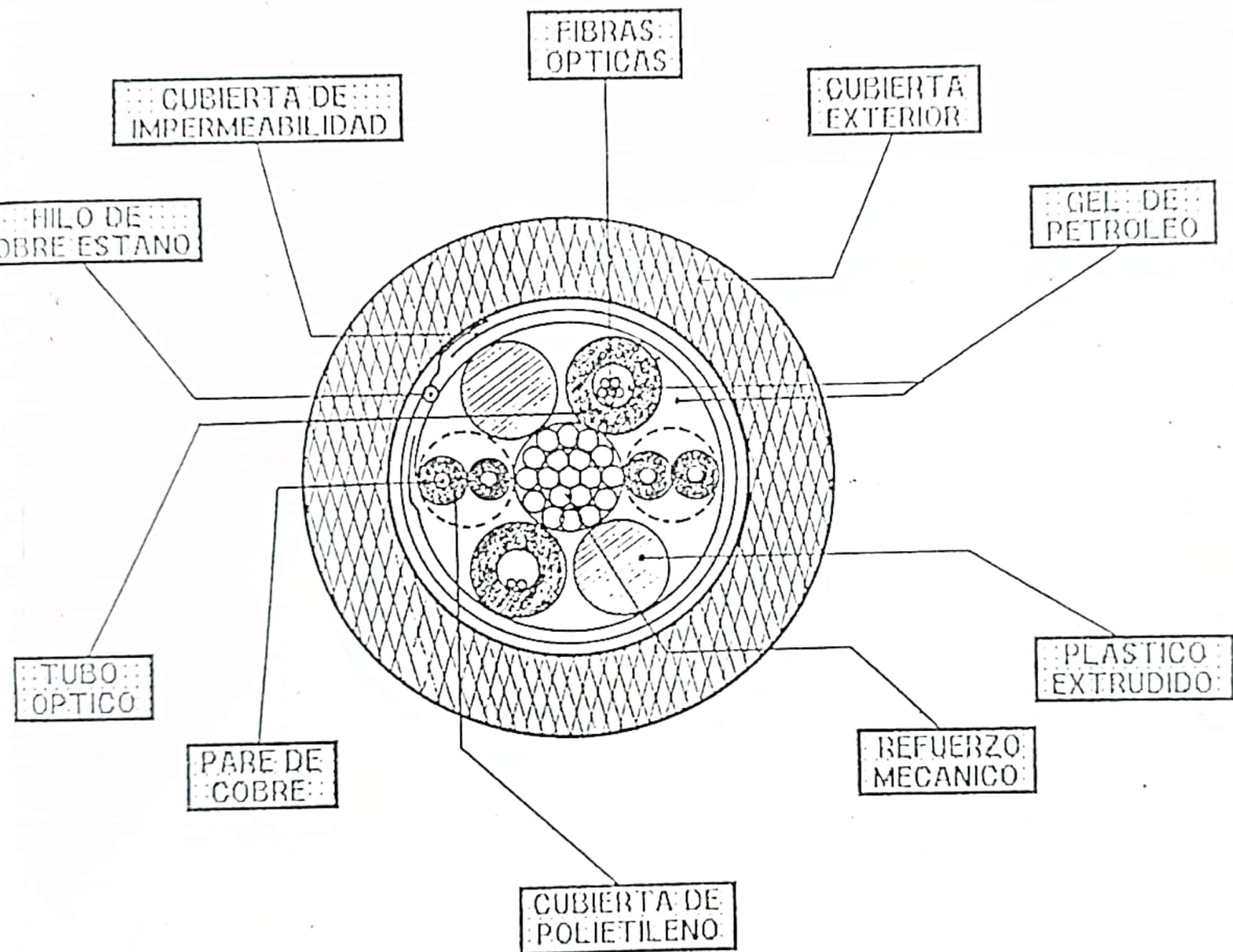
Fig. 10.2 CABLE DE FIBRA OPTICA UTILIZADO POR ALCATEL
