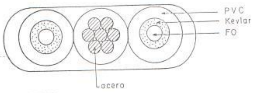
Fig. 2.3.3 DISTINTOS TIPOS DE CABLES CON FIBRAS OPTICAS
