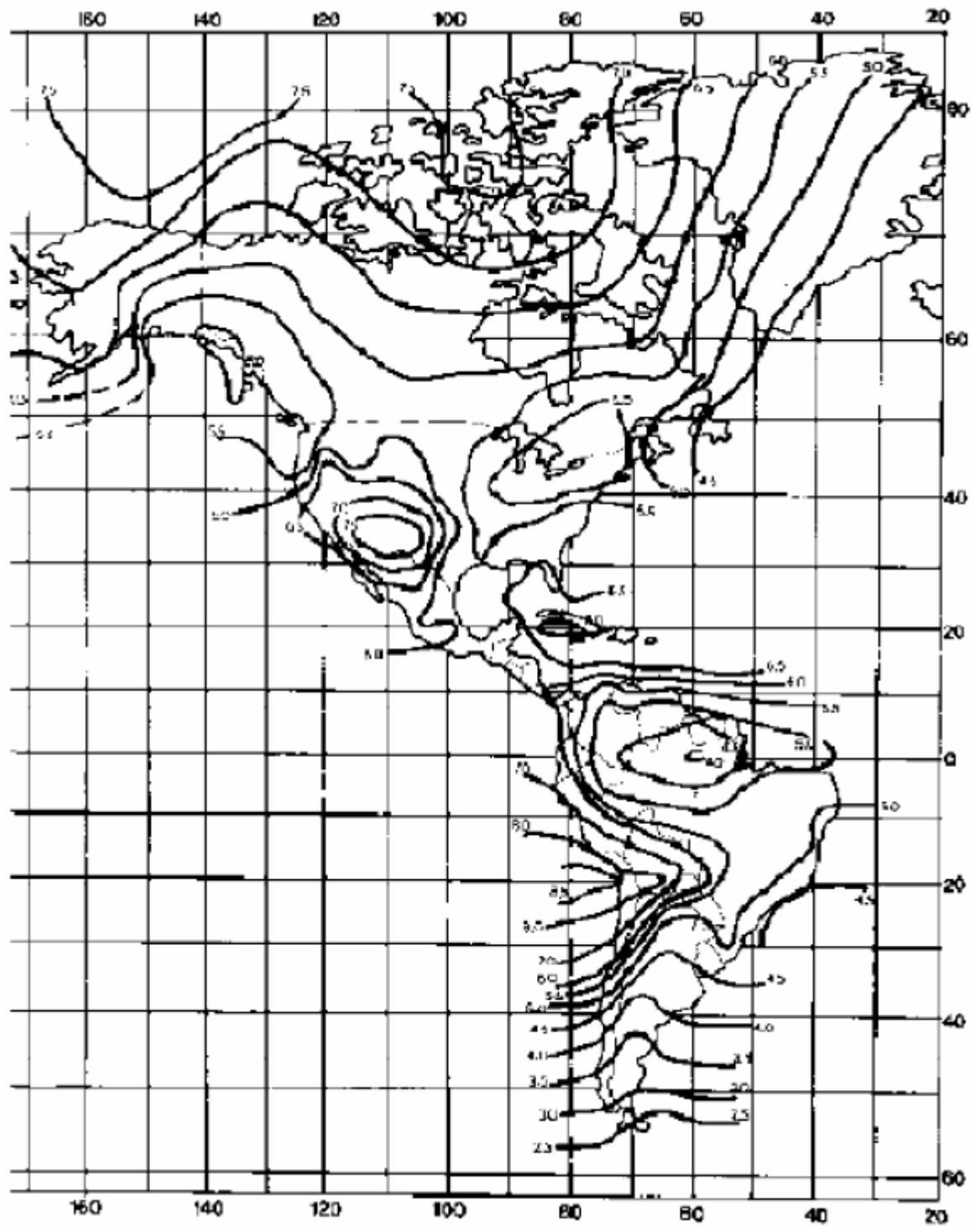
Fig. A2.2 Duración del Día Solar. Inclinación: Latitud +15^\circ Norte del Ecuador: Primavera Sur del Ecuador: Otoño
