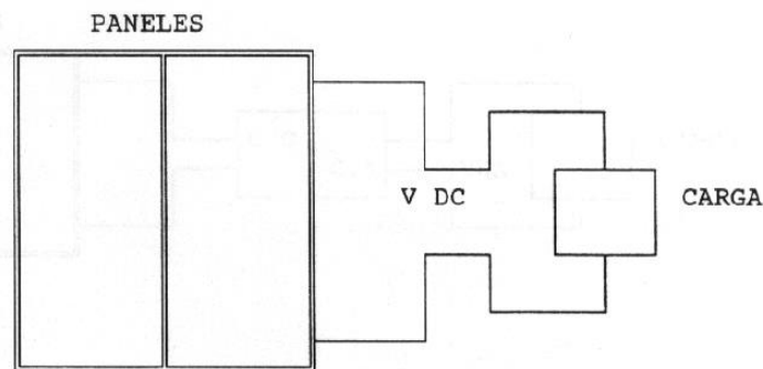
Figura 1.14.- Conexión típica de los paneles a la carga sin reguladores ni baterías
