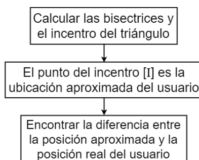
Figura 3.4: Tercera etapa del algoritmo
