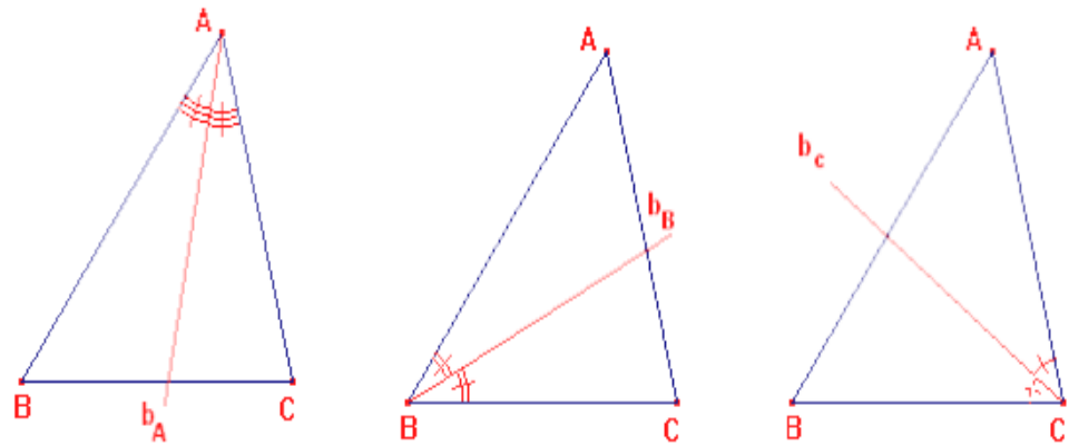
Figura 2.6: Triángulo ABC con sus bisectrices para cada ángulo [7].
