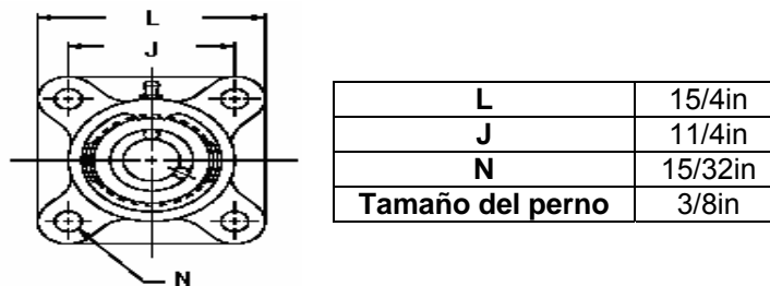
FIGURA 3.15. DIMENSIONES NOMINALES DE LA CHUMACERA.
