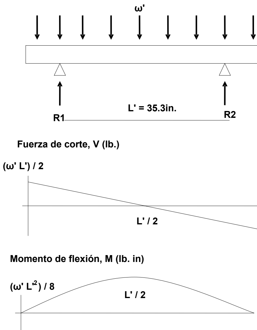
FIGURA 3.5. GRÁFICAS DE CARGA, CORTE Y MOMENTO.
