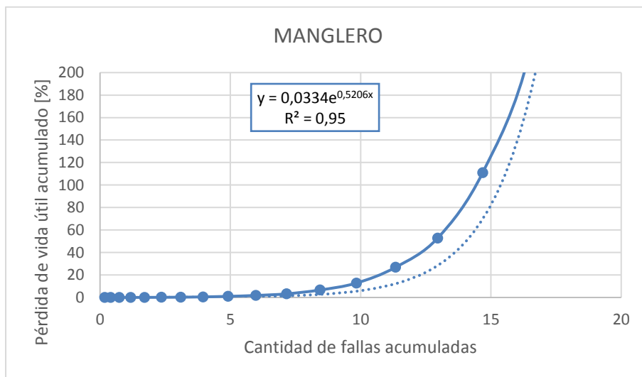
Figura 3.6: S/E Manglero Porcentaje acumulado de pérdida de vida útil en función de la cantidad de fallas acumuladas
