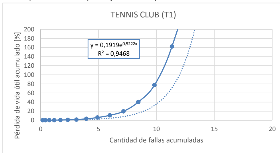
Figura 3.4: S/E Tennis Club (T1) Porcentaje acumulado de pérdida de vida útil en función de la cantidad de fallas acumuladas
