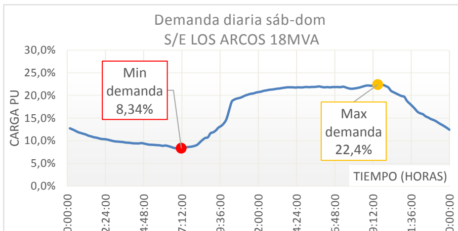
Figura 2.4: Demanda diaria sáb-dom S/E LOS ARCOS 18 MVA
