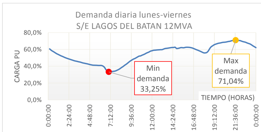
Figura 2.6: Demanda diaria lunes-viernes S/E LAGOS DEL BATÁN 12 MVA
