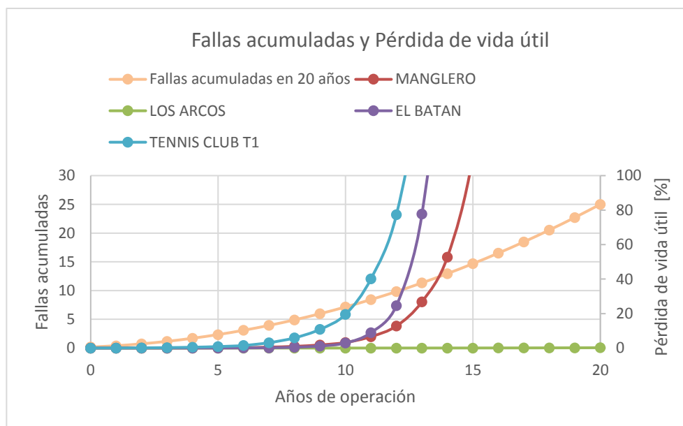
Figura 3.2: Fallas acumuladas y porcentaje de pérdida de vida útil acumulado anual para 20 años de operación
