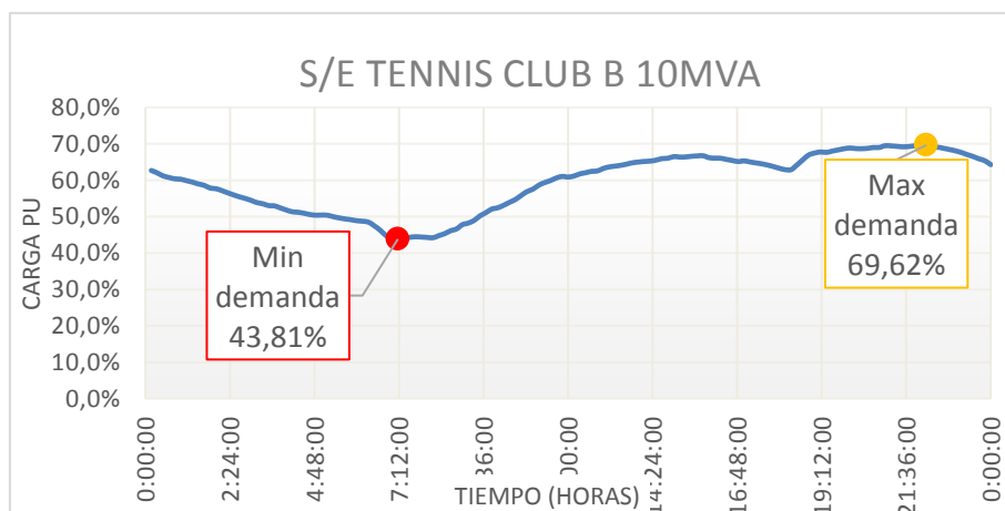
Figura B.6: Demanda fin de semana S/E Tennis Club B
