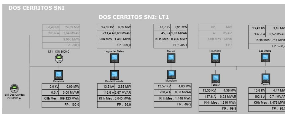
Figura 2.1: Unifilar del alimentador: Dos Cerritos SNI LT1. Obtenido del sistema de telemetría Guayas-Los Ríos.
