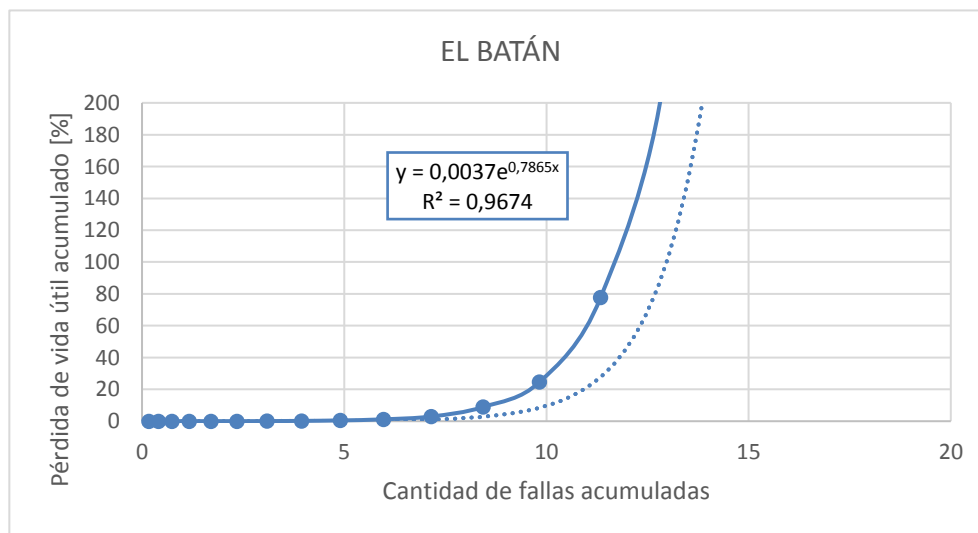
Figura 3.3: S/E El Batán Porcentaje acumulado de pérdida de vida útil en función de la cantidad de fallas acumuladas
