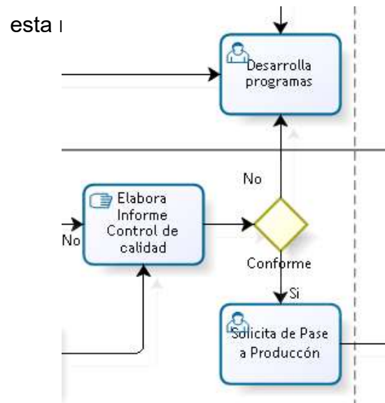
Figura 4.28: Validar Certificación
