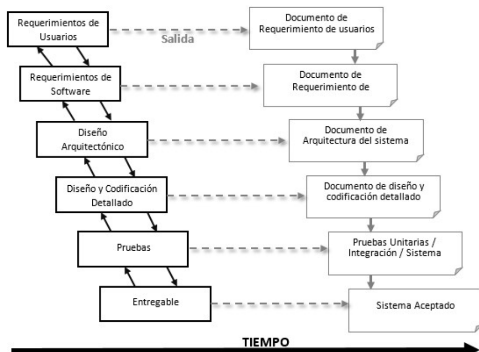
Figura 2.3: Metodología Clásica – Modelo en Cascada [11]
