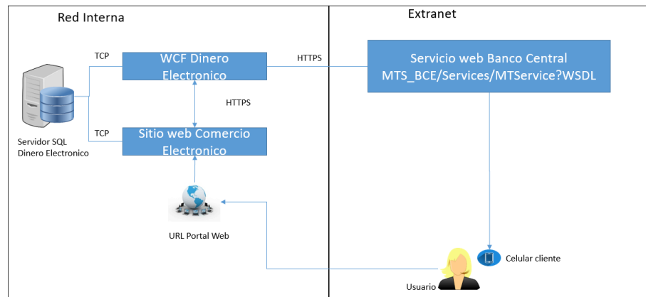
Figura 4.7 Diagrama de Arquitectura API Botón de pago dinero electrónico
